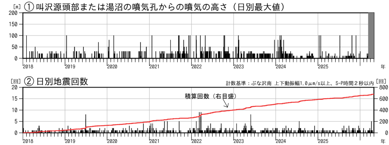
図2 秋田焼山 火山活動経過図（2018年1月～2026年4月）
