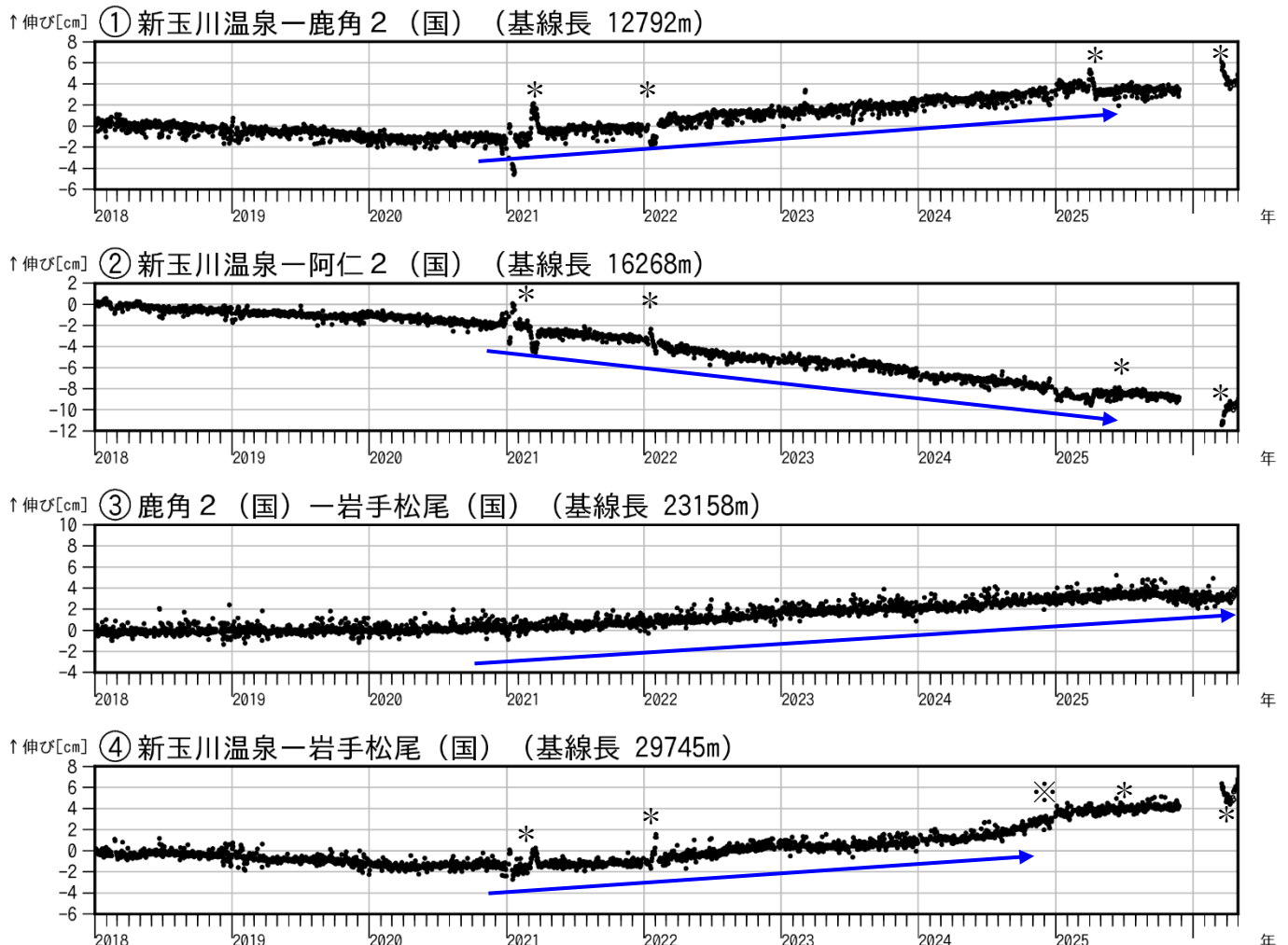
図3 秋田焼山 GNSS 基線長変化図（2018年1月～2026年4月）
