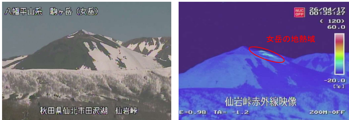
図1 秋田駒ヶ岳 女岳周辺の状況（4月19日）と地表面温度分布の状況（4月17日）
