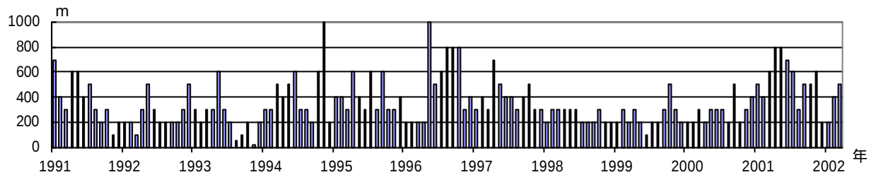
浅間山 月別最大噴煙高度*（1991年1月1日～2002年3月31日）
