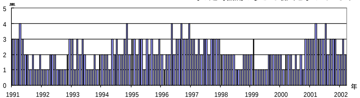
浅間山 月別最大噴煙量*（1991年1月1日～2002年3月31日）
