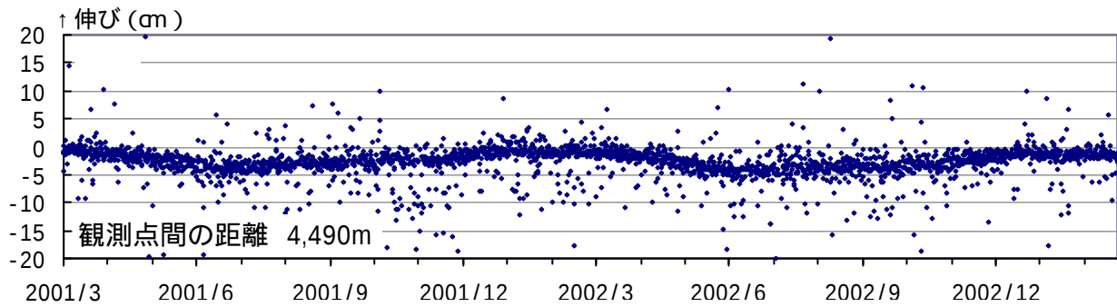
図 3 伊豆東部火山群 GPS 観測結果 (2001 年 3 月 1 日 ~ 2003 年 2 月 28 日) 大崎 - 伊東市 基線長
