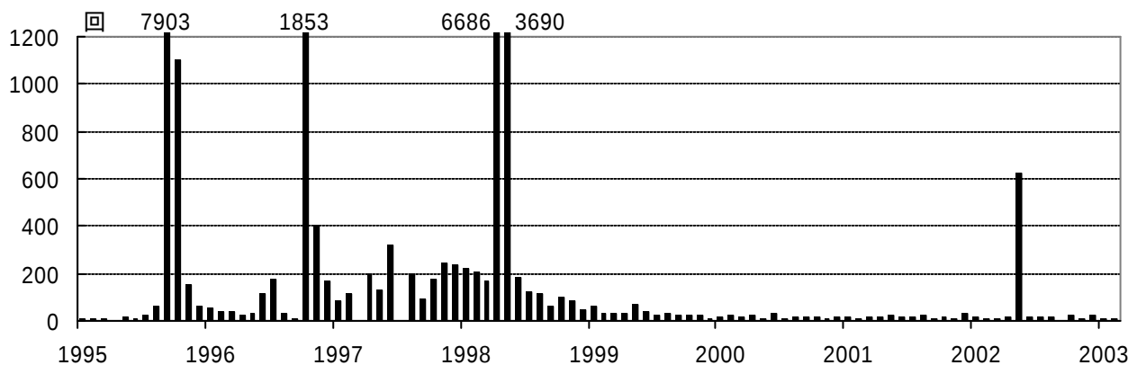
図 2 伊豆東部火山群 火山性地震月別回数（1995 年 1 月～2003 年 2 月）
