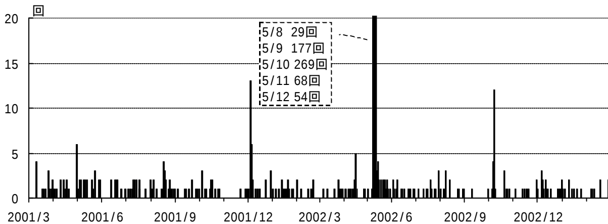
図 1 伊豆東部火山群 火山性地震日別回数 （2001 年 3 月 1 日～2003 年 2 月 28 日）
