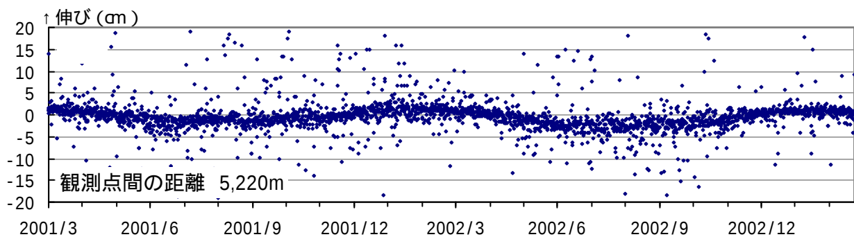
図 4 伊豆東部火山群 GPS 観測結果 (2001 年 3 月 1 日 ~ 2003 年 2 月 28 日) 大崎 - 新井 基線長
