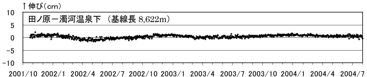
図2 御嶽山 GPS 観測結果(基線長変化)（2001年10月23日～2004年7月31日）
