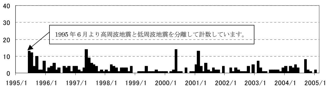
図 1 富士山 高周波地震月別回数(1995 年 6 月～2005 年 2 月)
