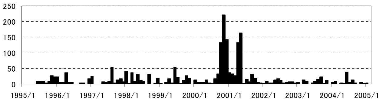
図 2 富士山 低周波地震月別回数(1995 年 6 月～2005 年 2 月)
