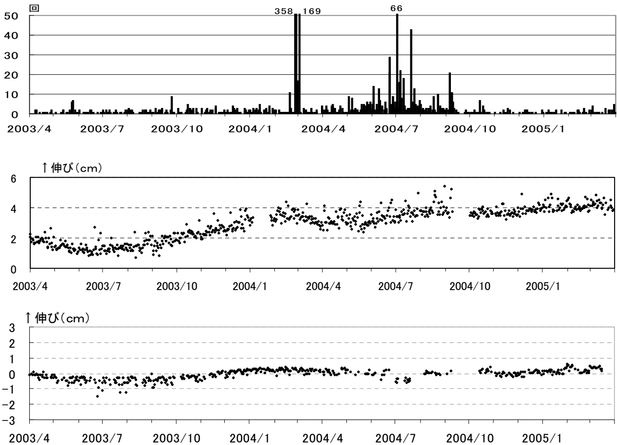
図5 伊豆大島 最近2年間（2003 年 3 月～2005 年 3 月）の活動 上：地震回数 中：①大島北西外輪～差木地奥山 GPS 観測 下：光波距離計（津倍付～神達）観測
