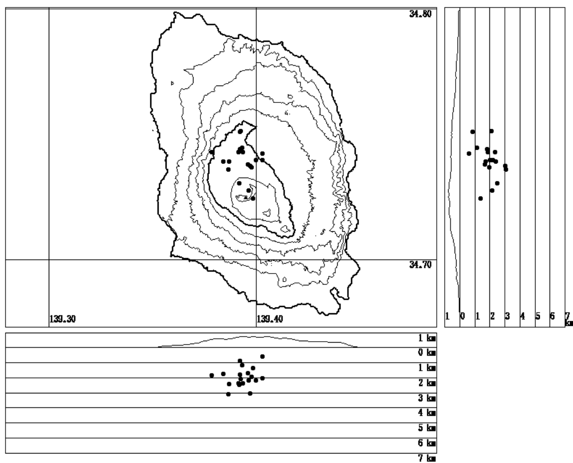
図2 伊豆大島 2005 年 3 月の地震活動
