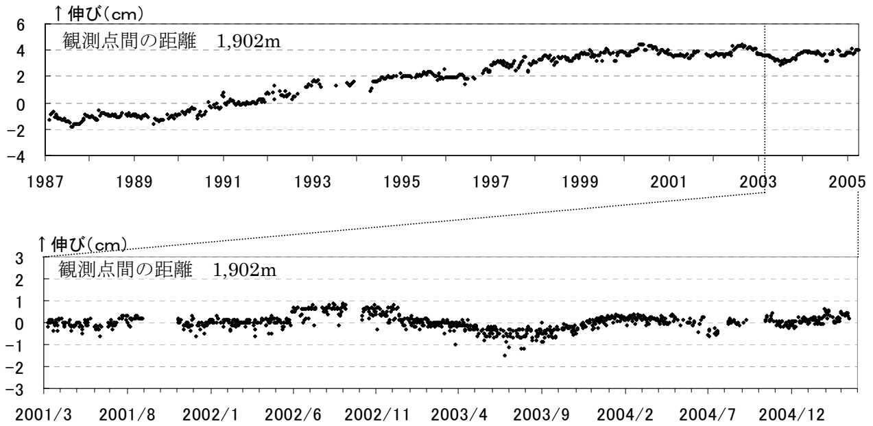
図4 伊豆大島 光波距離計（津倍付～神達）斜距離変化 上：旬平均値（1987 年 1 月～2005 年 3 月） 下：日平均値（2001 年 3 月 1 日～2005 年 3 月 31 日）
