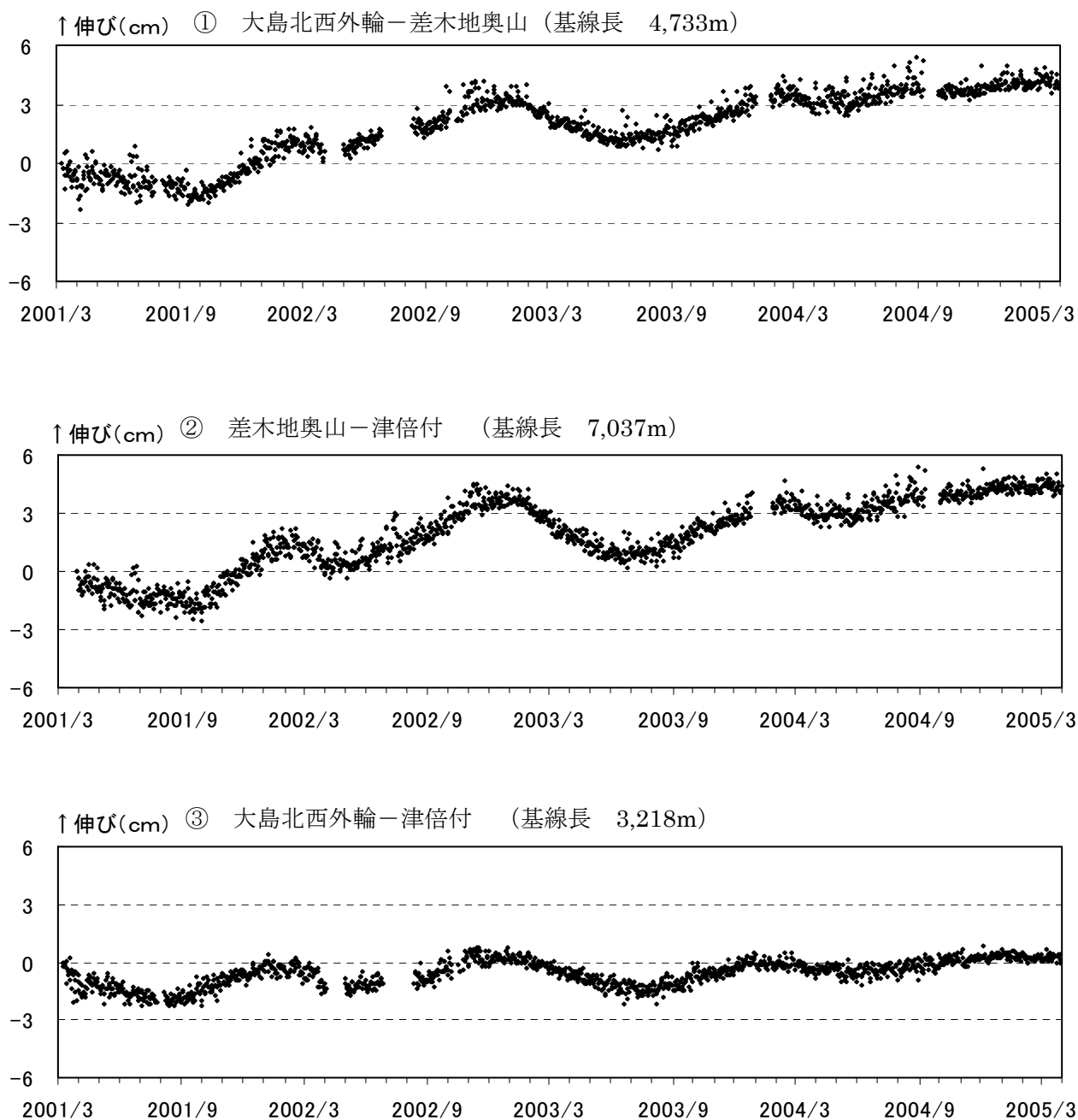
図 3 伊豆大島 GPS 観測結果（基線長変化）（2001 年 3 月 7 日～2005 年 3 月 31 日）
