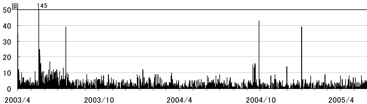
図 1 御嶽山 日別地震回数（2003 年 4 月 1 日～2005 年 5 月 31 日）
