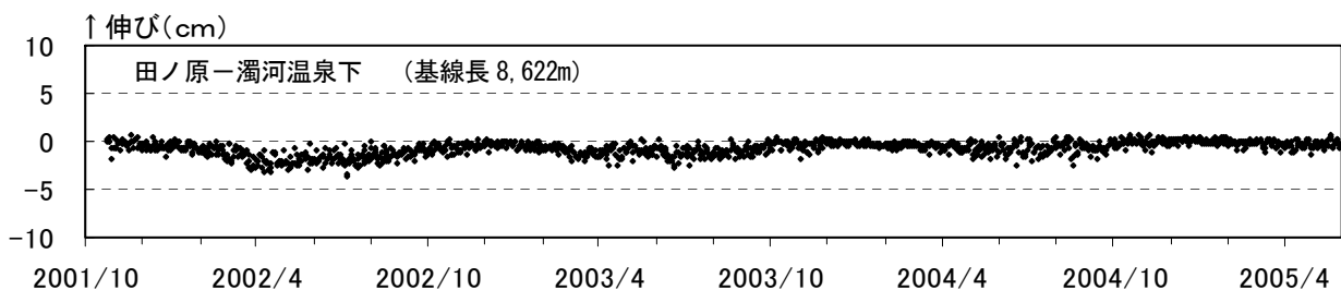
図 2 御嶽山の GPS 連続観測による基線長変化（2001 年 10 月 23 日～2005 年 5 月 31 日）
