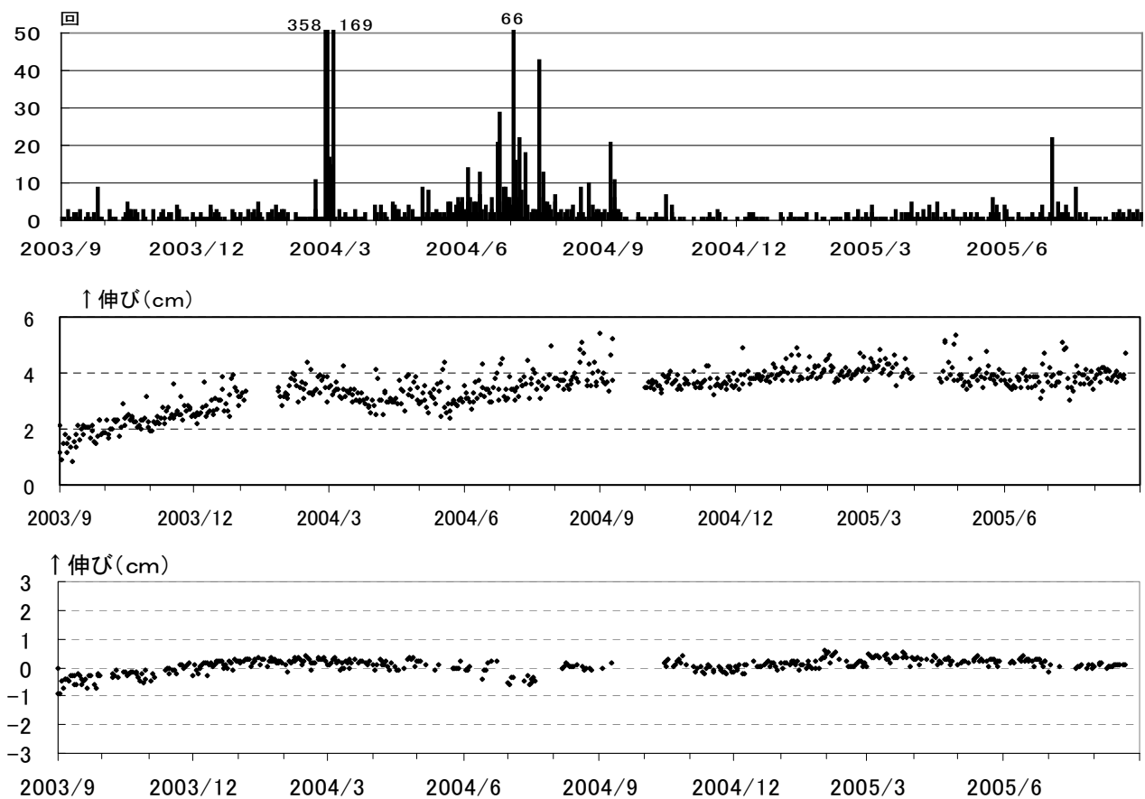
図5 伊豆大島 最近 2 年間（2003 年 9 月～2005 年 8 月）の活動 上：地震回数 中：①大島北西外輪～差木地奥山 GPS 観測 下：光波距離計（津倍付～神達）観測
