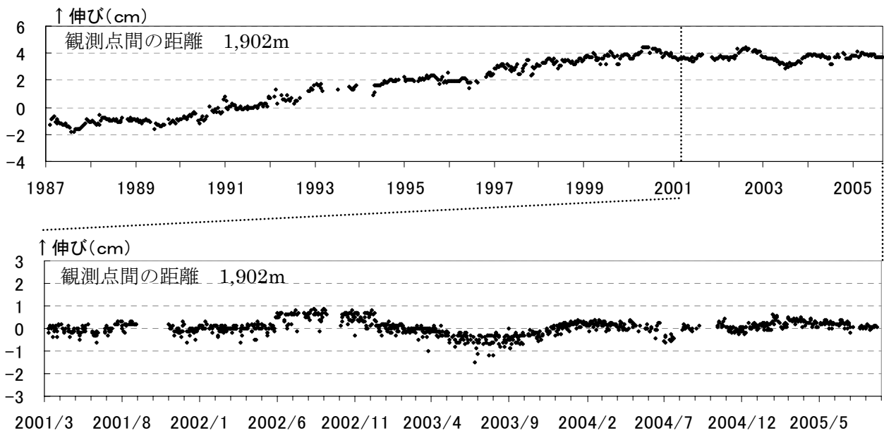
図4 伊豆大島 光波距離計（津倍付～神達）斜距離変化 上：旬平均値（1987 年 1 月～2005 年 8 月） 下：日平均値（2001 年 3 月 1 日～2005 年 8 月 31 日）
