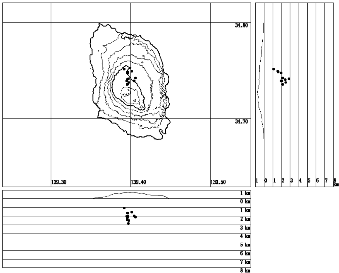
図 2 伊豆大島 2005 年 8 月の地震活動
