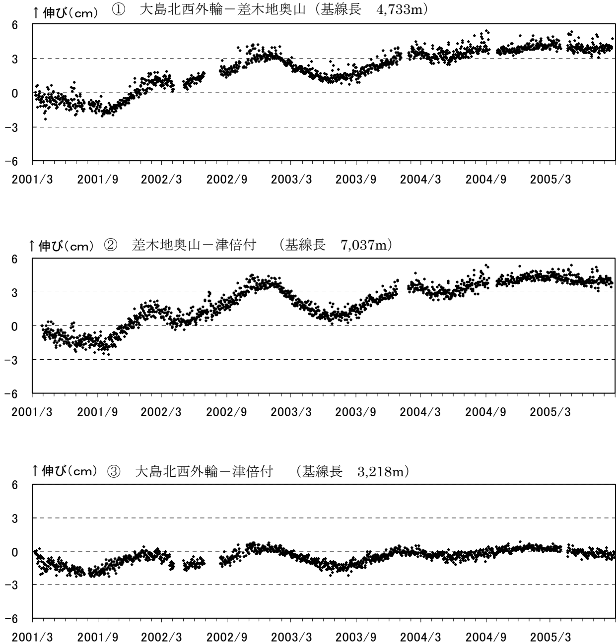
図 3 伊豆大島 GPS 観測結果（基線長変化）（2001 年 3 月 7 日～2005 年 8 月 31 日）
