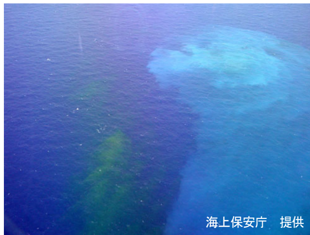
図 1 福德岡ノ場 変色水の状況その 1（2005 年 11 月 28 日）
