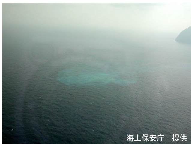
図 2 福德岡ノ場 変色水の状況その 2（2005 年 11 月 28 日）
