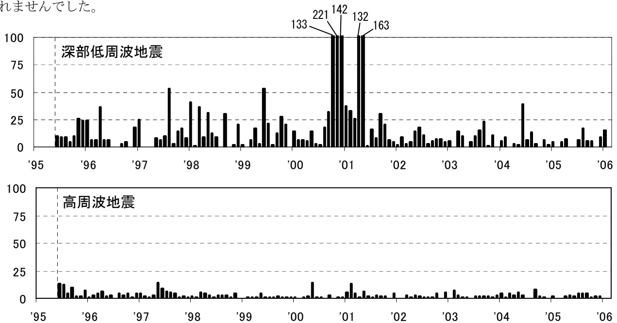
図1※ 富士山 月別地震回数（1995年6月～2006年1月）
