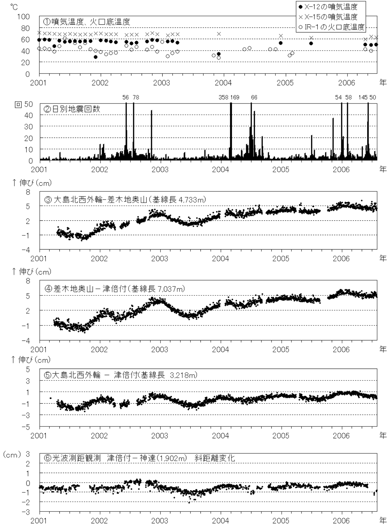
図5 伊豆大島 最近の火山活動経過図（2001年1月～2006年7月）
