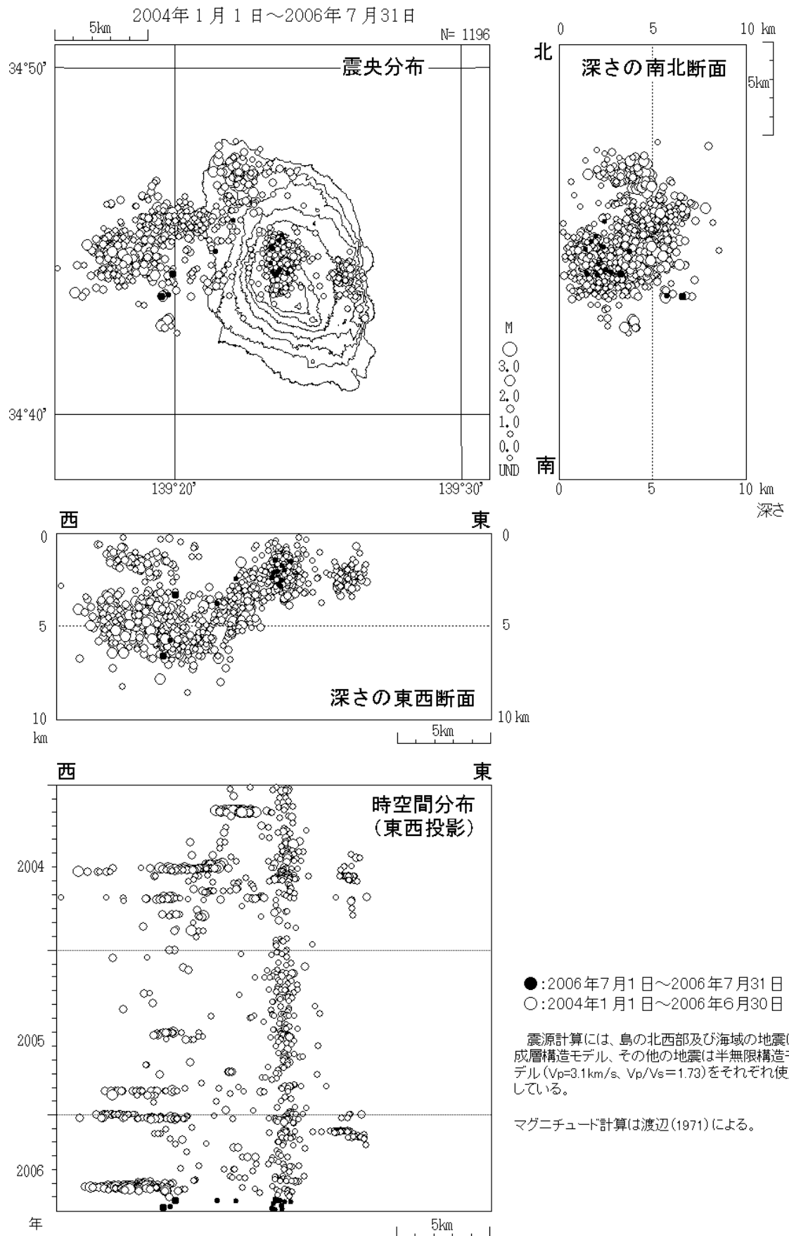
図 6※ 伊豆大島 震源分布(2004 年 1 月 1 日～2006 年 7 月 31 日)
