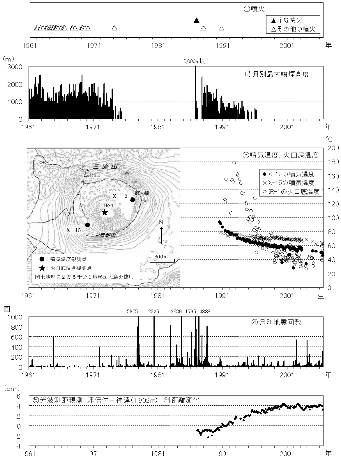
図4 伊豆大島 長期間の火山活動経過図（1961 年 1 月～2006 年 7 月）
