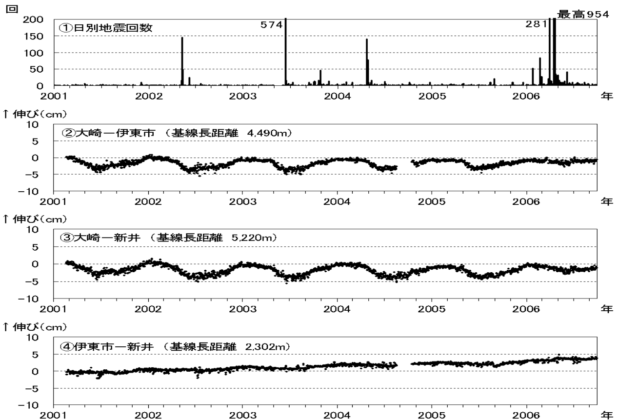
図2 伊豆東部火山群 鎌田地震観測点（図3右図）で観測した日別地震回数とGPS連続観測による基線長変化（2001年1月～2006年9月）
