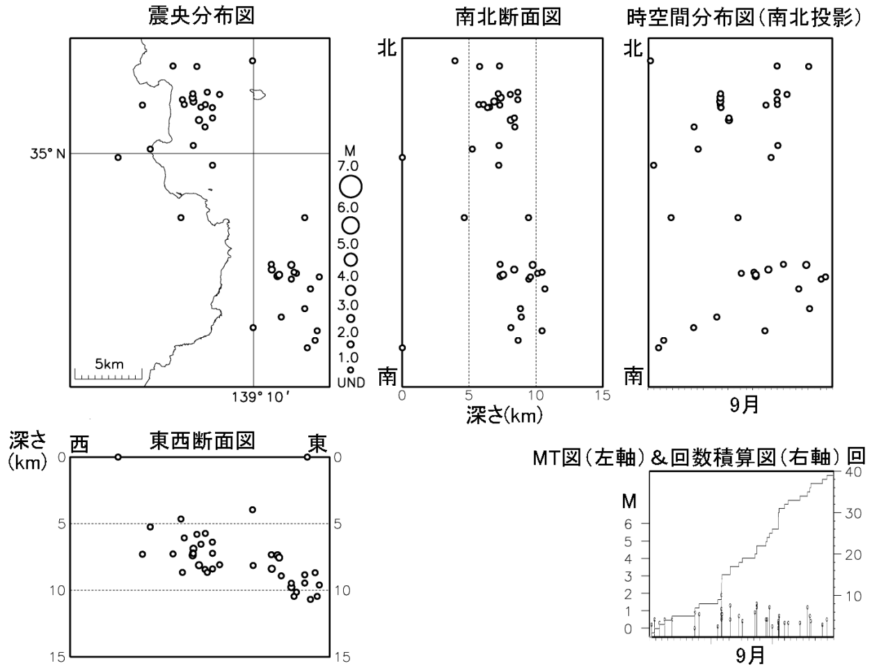
図 1 ※ 9 月の地震活動経過（2006 年 9 月 1 日～9 月 30 日、マグニチュード 1) は暫定値）
