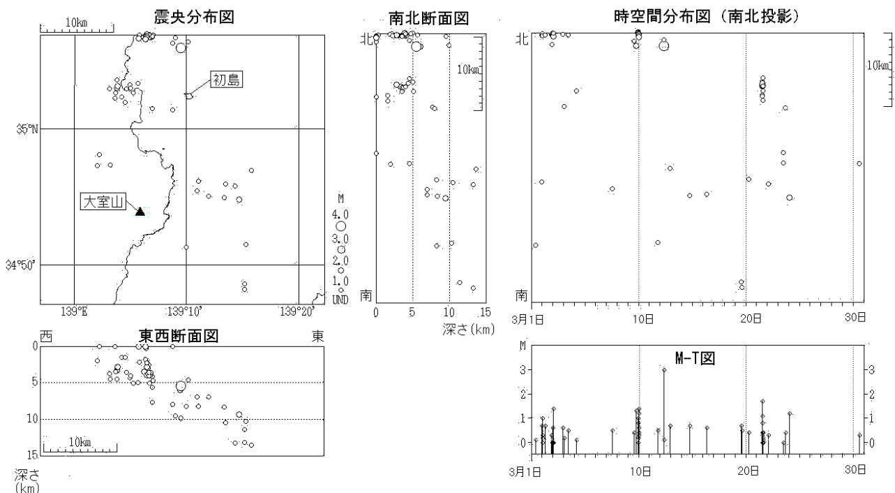
図1※ 伊豆東部火山群 地震活動経過図（2007年3月1日～3月31日）
