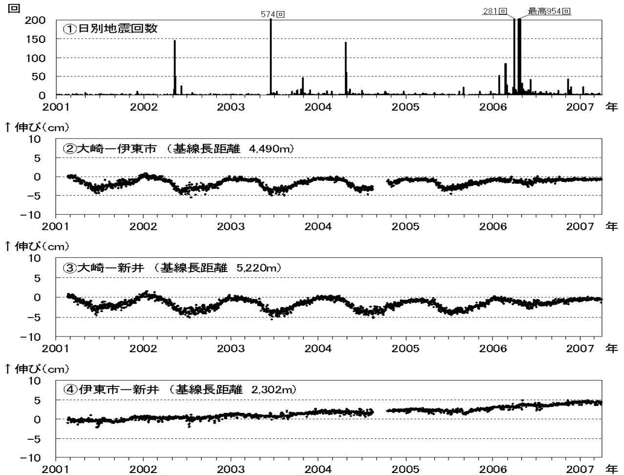
図 2 伊豆東部火山群 最近の火山活動の推移（2001 年 1 月～2007 年 3 月）
