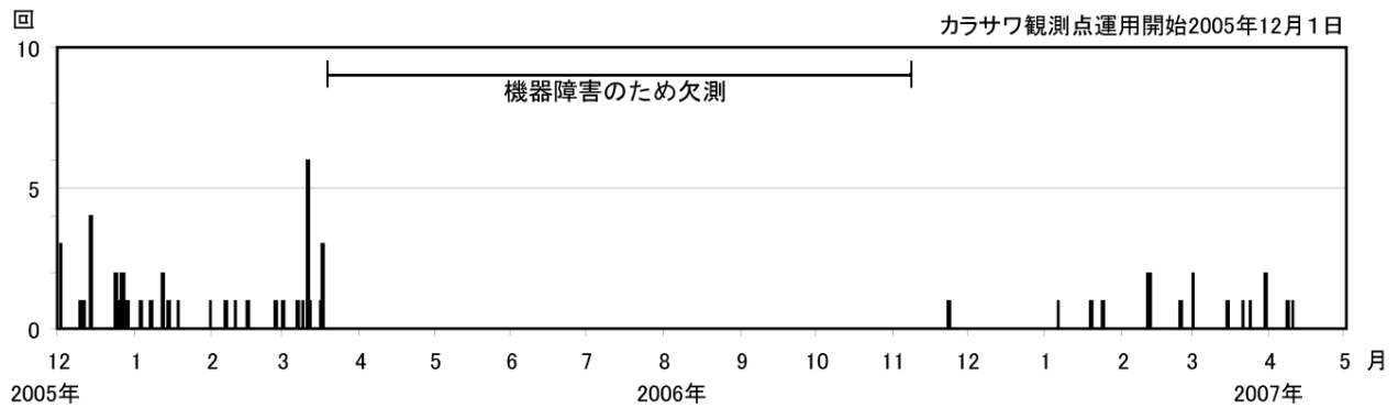
図2 新潟焼山 日別地震回数（2005年12月1日～2007年4月30日）
