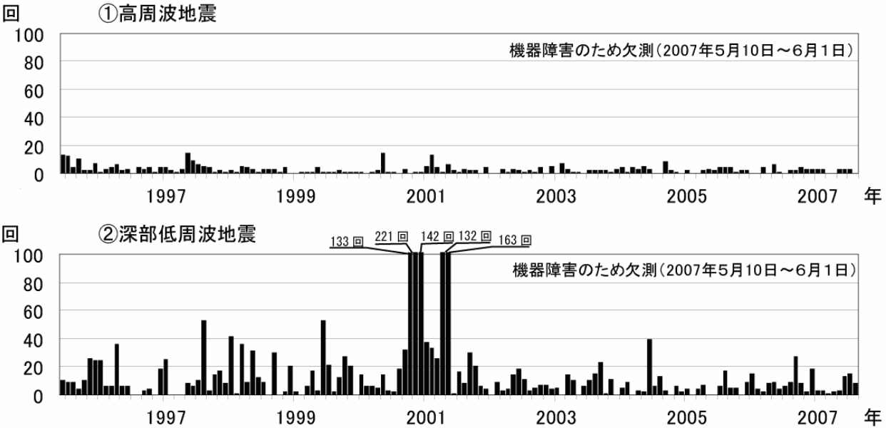
図 1 富士山 月別地震回数(1995 年 6 月～2007 年 8 月)
