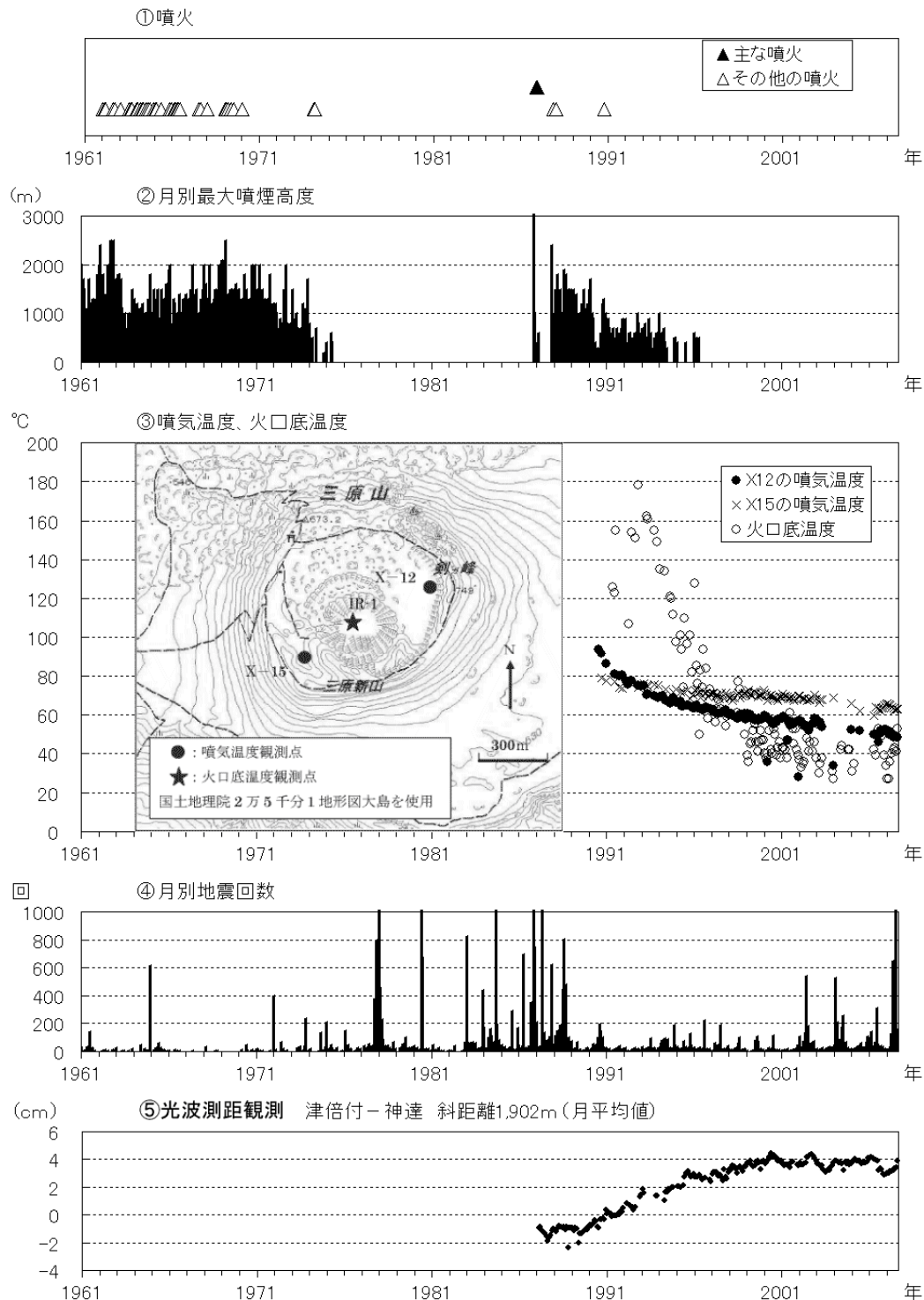
図4 伊豆大島 長期間の火山活動経過図（1961年1月～2007年8月）
