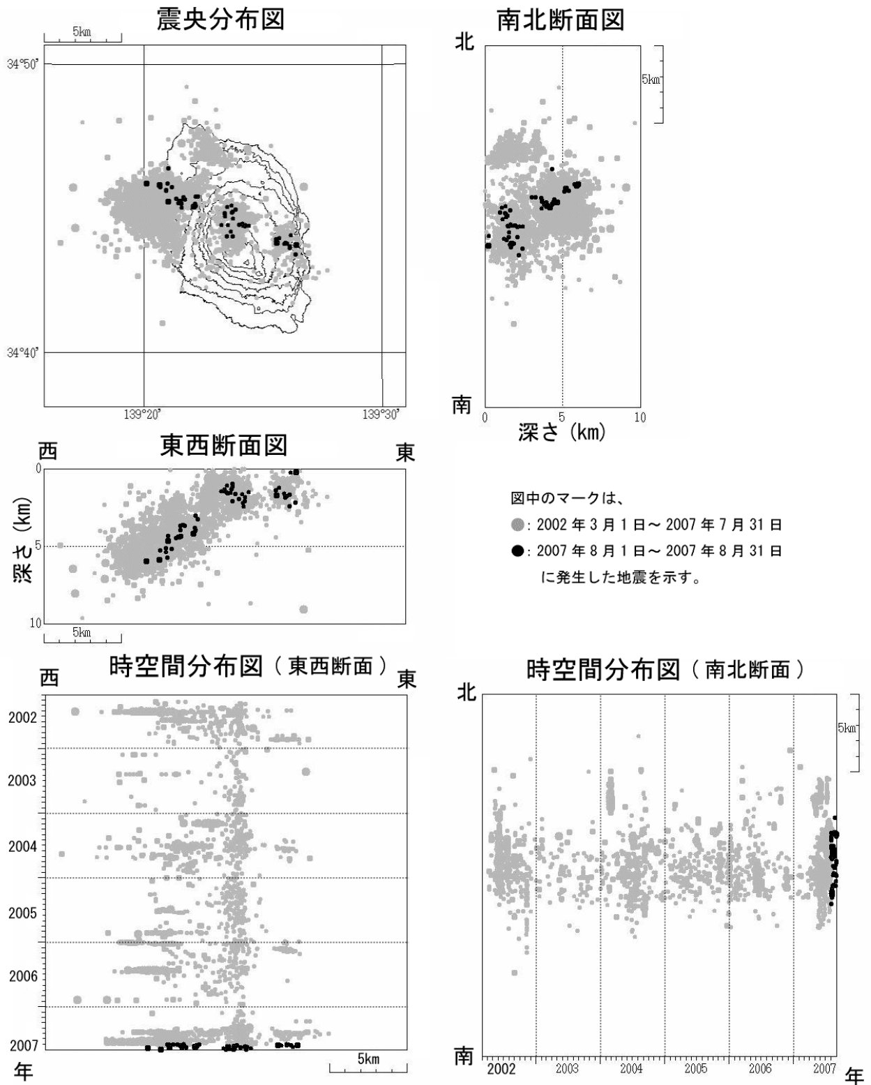
図 6 伊豆大島 震源分布図（2002 年 3 月 1 日～2007 年 8 月 31 日）
