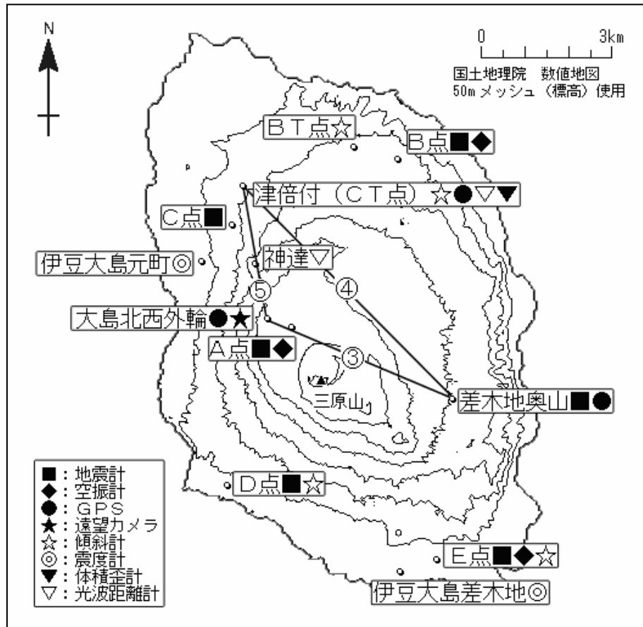
図 7 伊豆大島 気象庁の観測点配置図（小さな白丸は観測点位置を示しています） 図中の ~ は図 5 の GPS 基線 ~ に対応しています。
