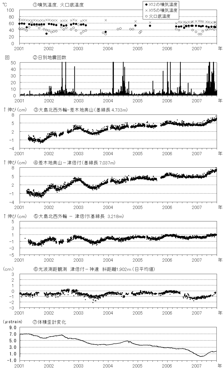
図 5 伊豆大島 最近の火山活動経過図（2001 年 1 月～2007 年 8 月）
