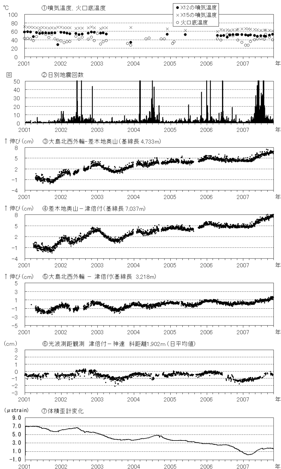
図5 伊豆大島 最近の火山活動経過図（2001年1月～2007年10月）
