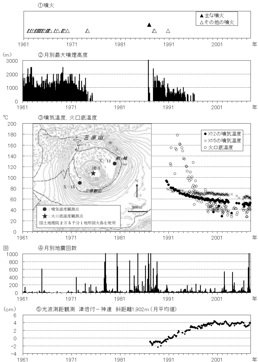
図4 伊豆大島 長期間の火山活動経過図（1961年1月～2007年10月）
