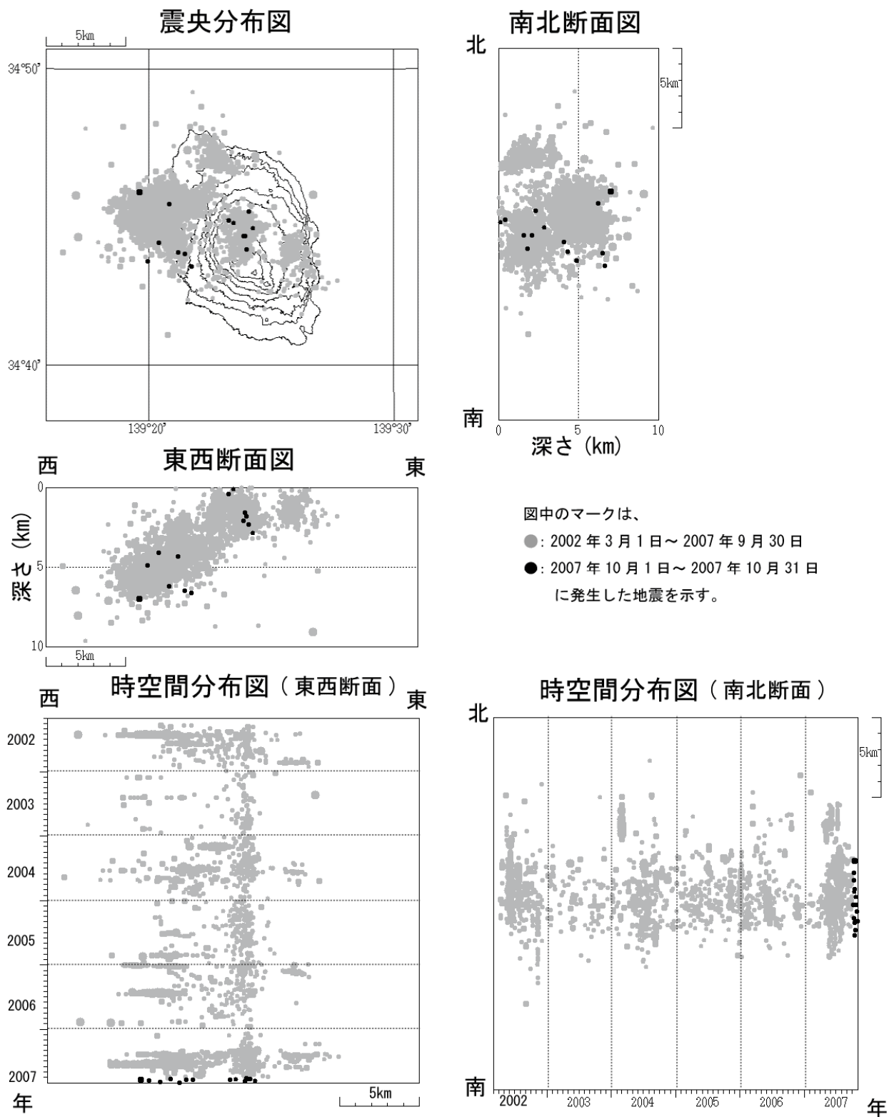
図 6※ 伊豆大島 震源分布図（2002 年 3 月 1 日～2007 年 10 月 31 日）
