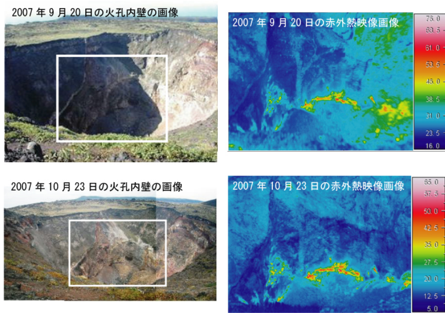
図 2 伊豆大島 中央火口北側内壁の状況（左）と地表面温度分布 1) （右） （左の写真の白枠部分が右の赤外熱映像撮影部分）
