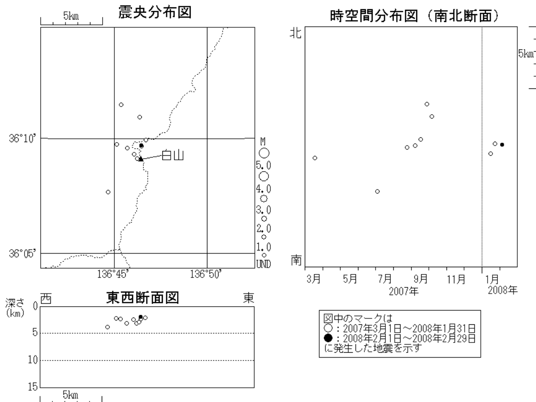
図 1 白山 山体周辺及びその周辺の地震活動（2007 年 3 月 1 日～2008 年 2 月 29 日）
