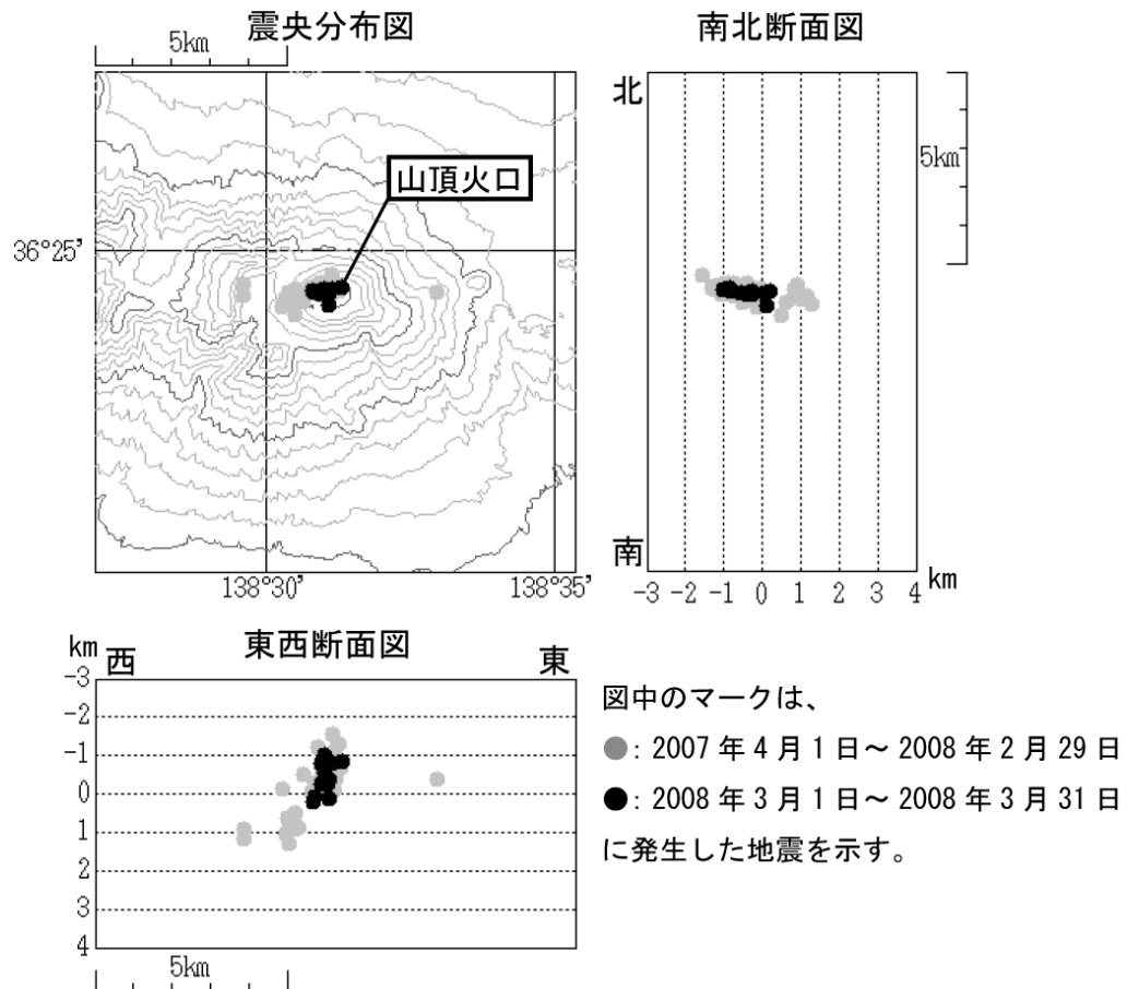
図 3※ 浅間山 火山性地震の震源分布（2007 年 4 月 1 日～2008 年 3 月 31 日）
