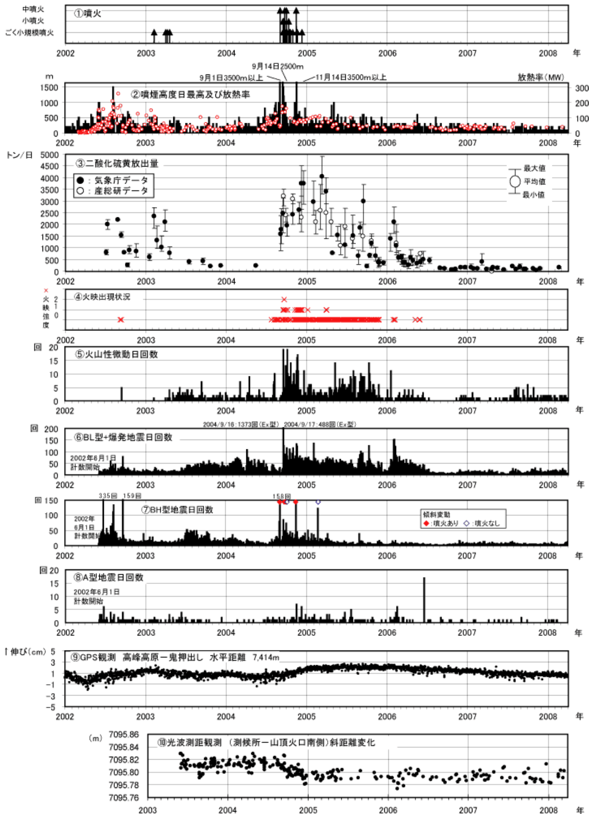
図 2※ 浅間山 最近の火山活動の推移（2002 年 1 月～2008 年 3 月）
