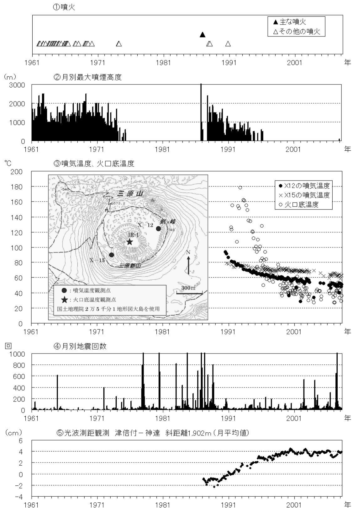
図4 伊豆大島 長期間の火山活動経過図（1961年1月～2008年3月）
