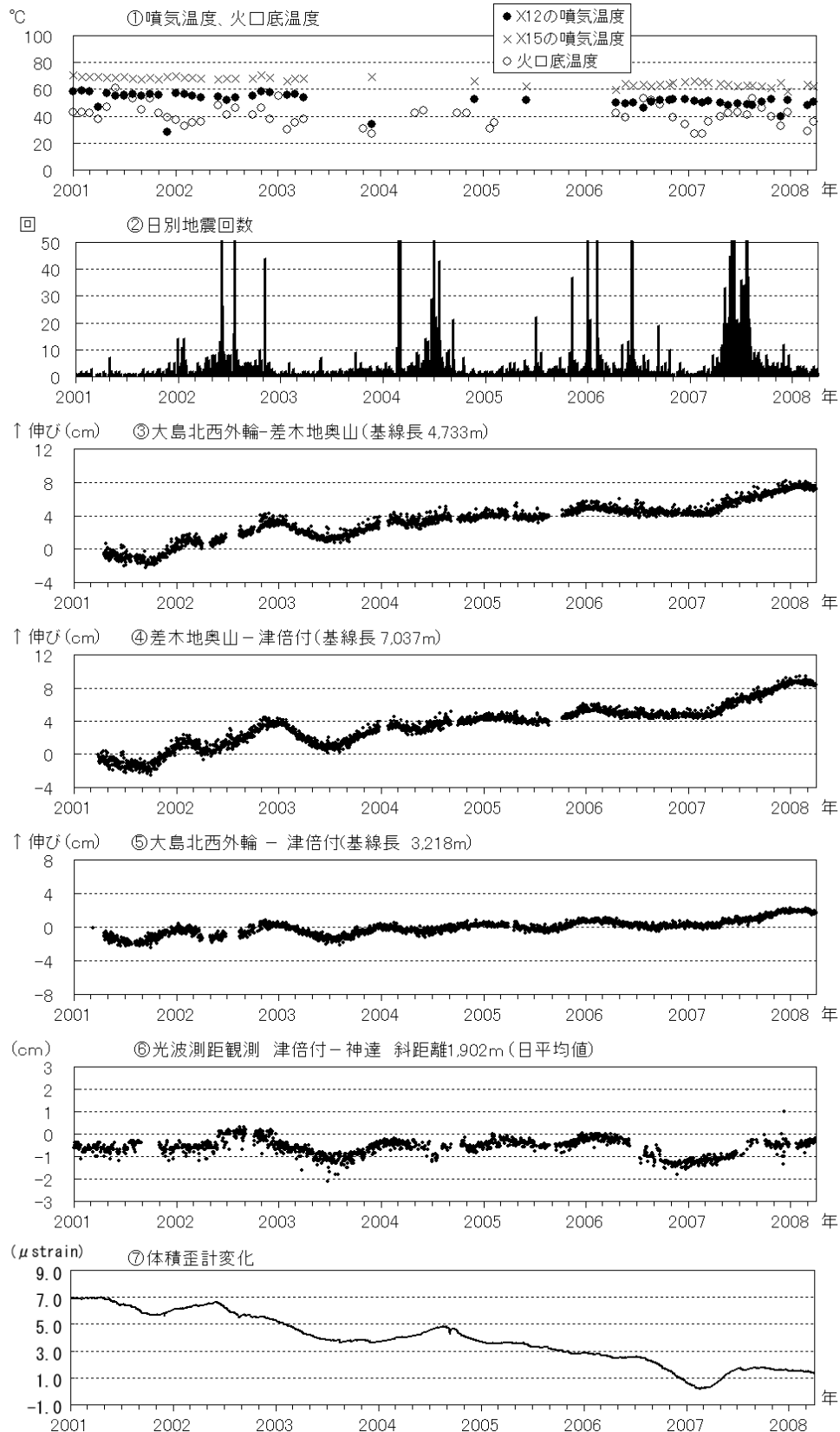
図 5 伊豆大島 最近の火山活動経過図（2001 年 1 月～2008 年 3 月）
