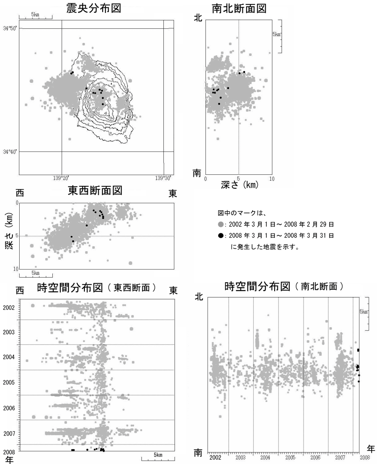
図 6※ 伊豆大島 震源分布図（2002 年 3 月 1 日～2008 年 3 月 31 日）
