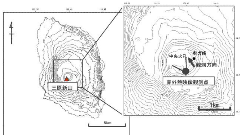
図3 伊豆大島 中央火口内の地表面温度分布 1) を測定した位置
