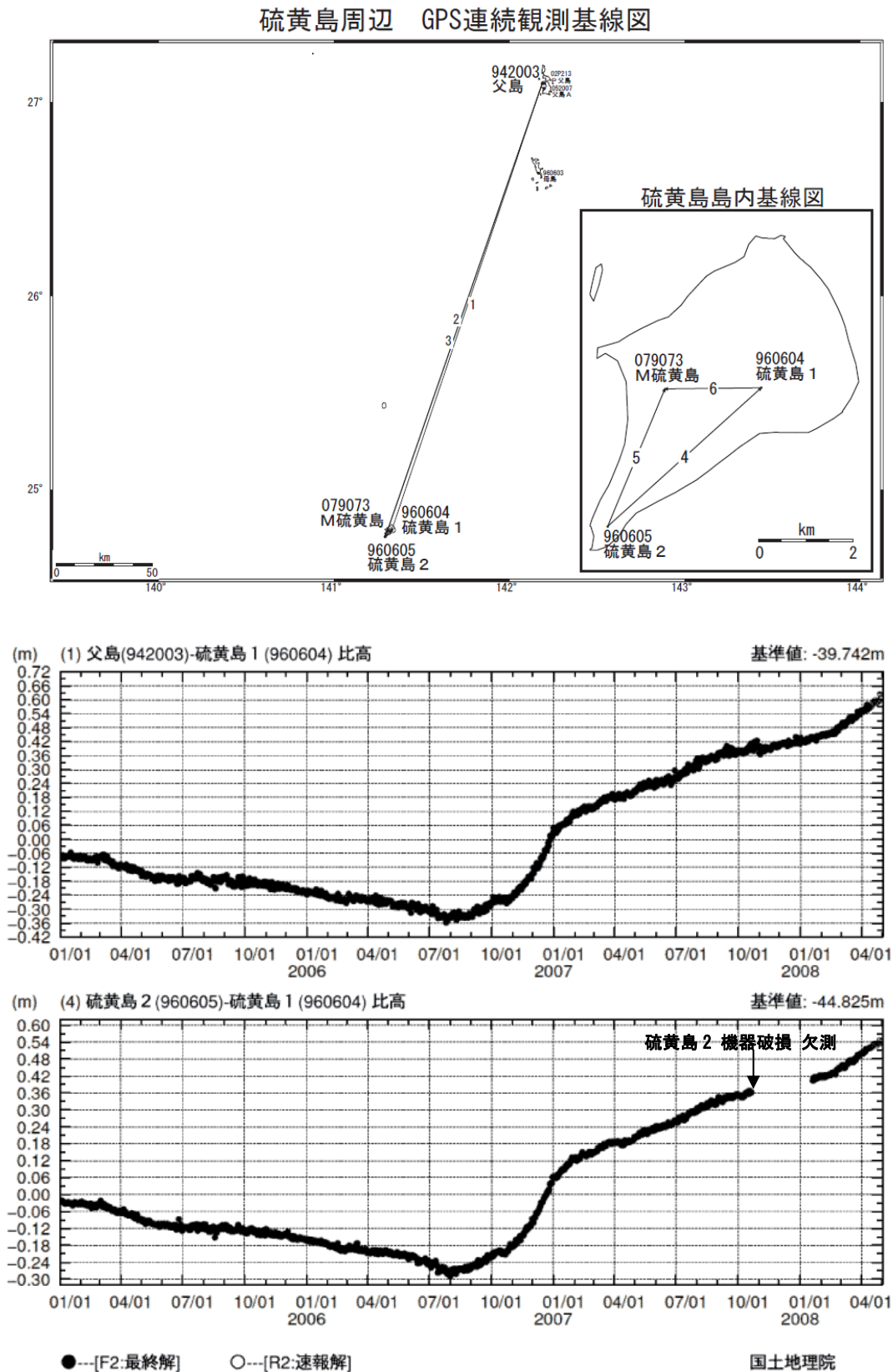
図 1 ※ 硫黄島 国土地理院による GPS 観測結果 1)
