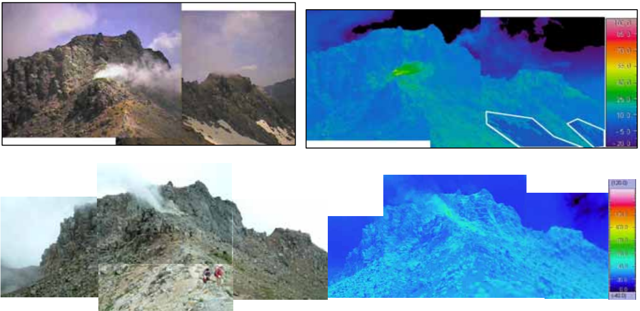
図2 焼岳 北峰南側斜面の地表面温度分布（撮影地点 図1の①） （上：2008年6月7日撮影、下：2003年7月26日撮影、白枠内は残雪）
