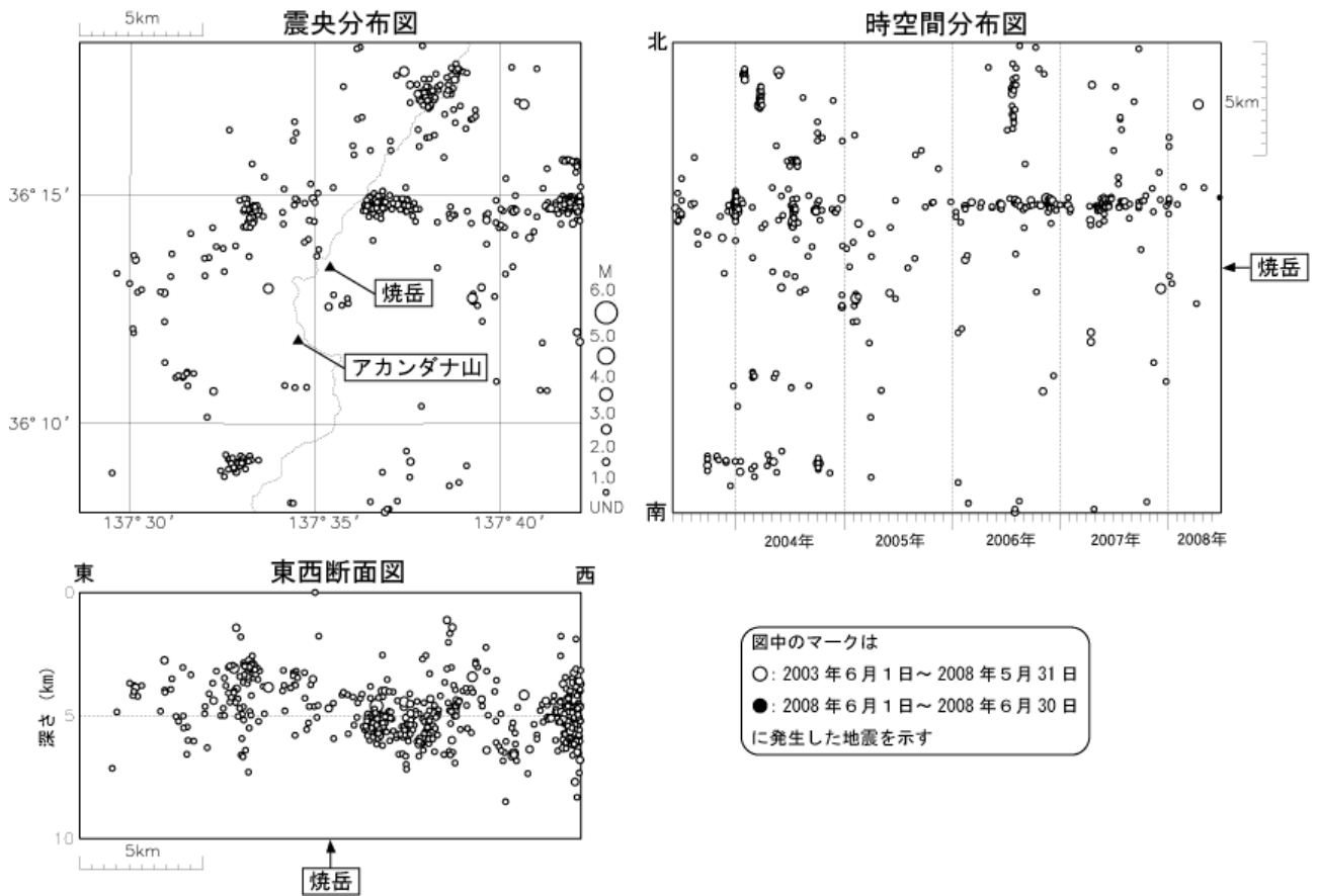
図 6 ※ 焼岳 山体及びその周辺の地震活動（2003 年 6 月 1 日～2008 年 6 月 30 日） M（マグニチュード）は地震の規模を表します。図中の震源要素は一部暫定値で、後日変更することがあります。
