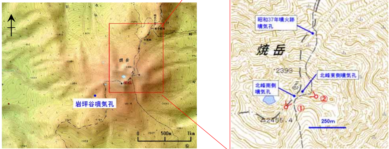
図 1 焼岳 噴気孔の位置および赤外熱映像撮影位置
