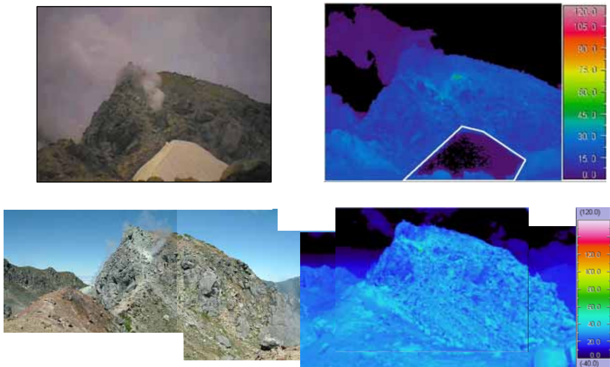
図3 焼岳 北峰東側斜面の地表面温度分布（撮影地点 図1の②） （上：2008年6月7日撮影、下：2003年7月26日撮影、白枠内は残雪）
