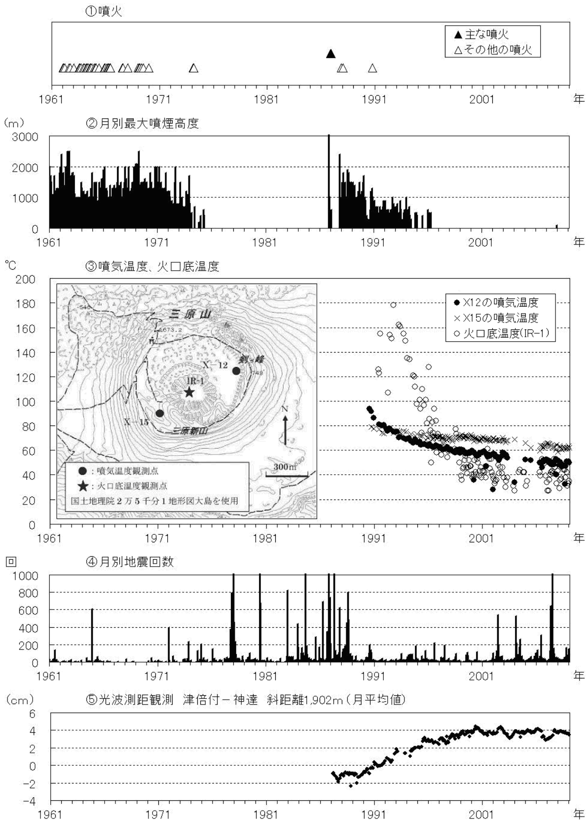
図4 伊豆大島 長期間の火山活動経過図（1961年1月～2009年1月）
