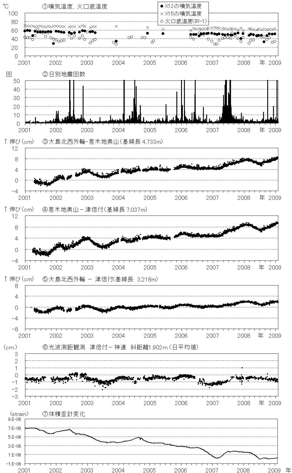
図5 伊豆大島 最近の火山活動経過図(2001年1月～2009年1月)
