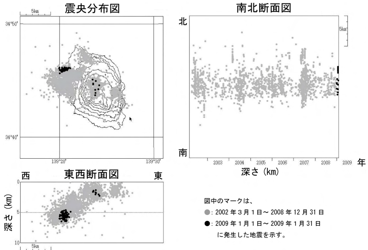
図 6※ 伊豆大島 震源分布図（2002 年 3 月 1 日～2009 年 1 月 31 日）
