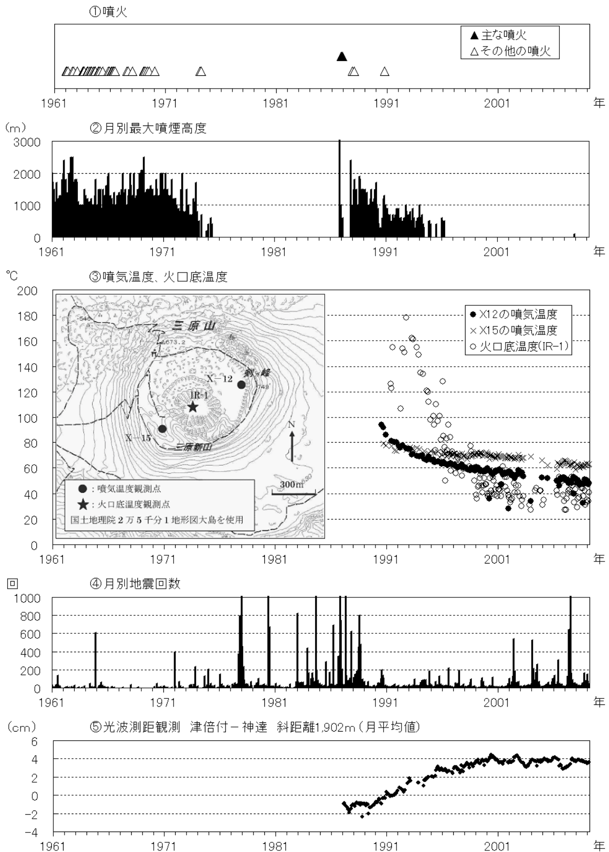
図4 伊豆大島 長期間の火山活動経過図（1961年1月～2009年3月）
