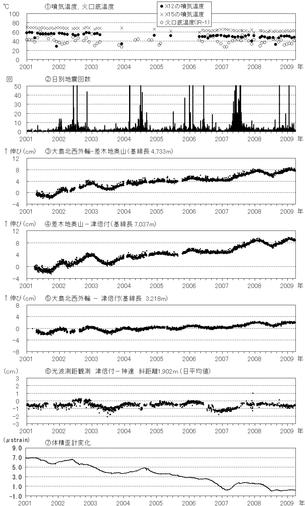
図 5 伊豆大島 最近の火山活動経過図（2001 年 1 月～2009 年 3 月）
