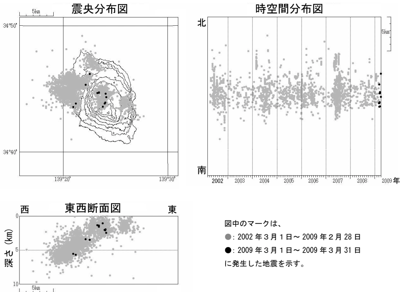
図 6 伊豆大島 震源分布図（2002 年 3 月 1 日～2009 年 3 月 31 日）
