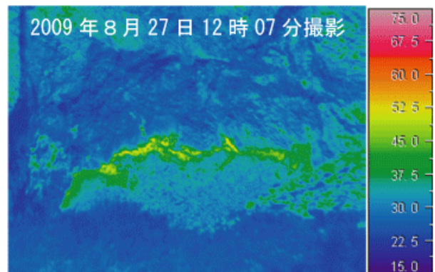
図2 伊豆大島 中央火口内の状況（左）と地表面温度分布 1) （右） （左の写真の白枠部分が右の赤外熱映像撮影部分）
