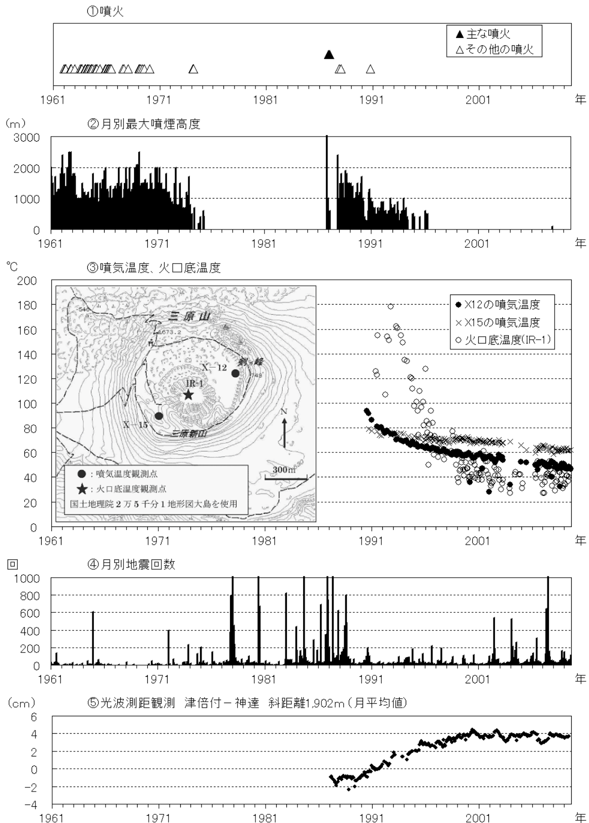
図 4 伊豆大島 長期間の火山活動経過図（1961 年 1 月～2009 年 8 月）
