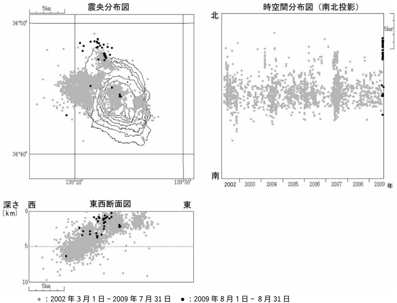
図 6 伊豆大島 震源分布図（2002 年 3 月 1 日 ~ 2009 年 8 月 31 日）
