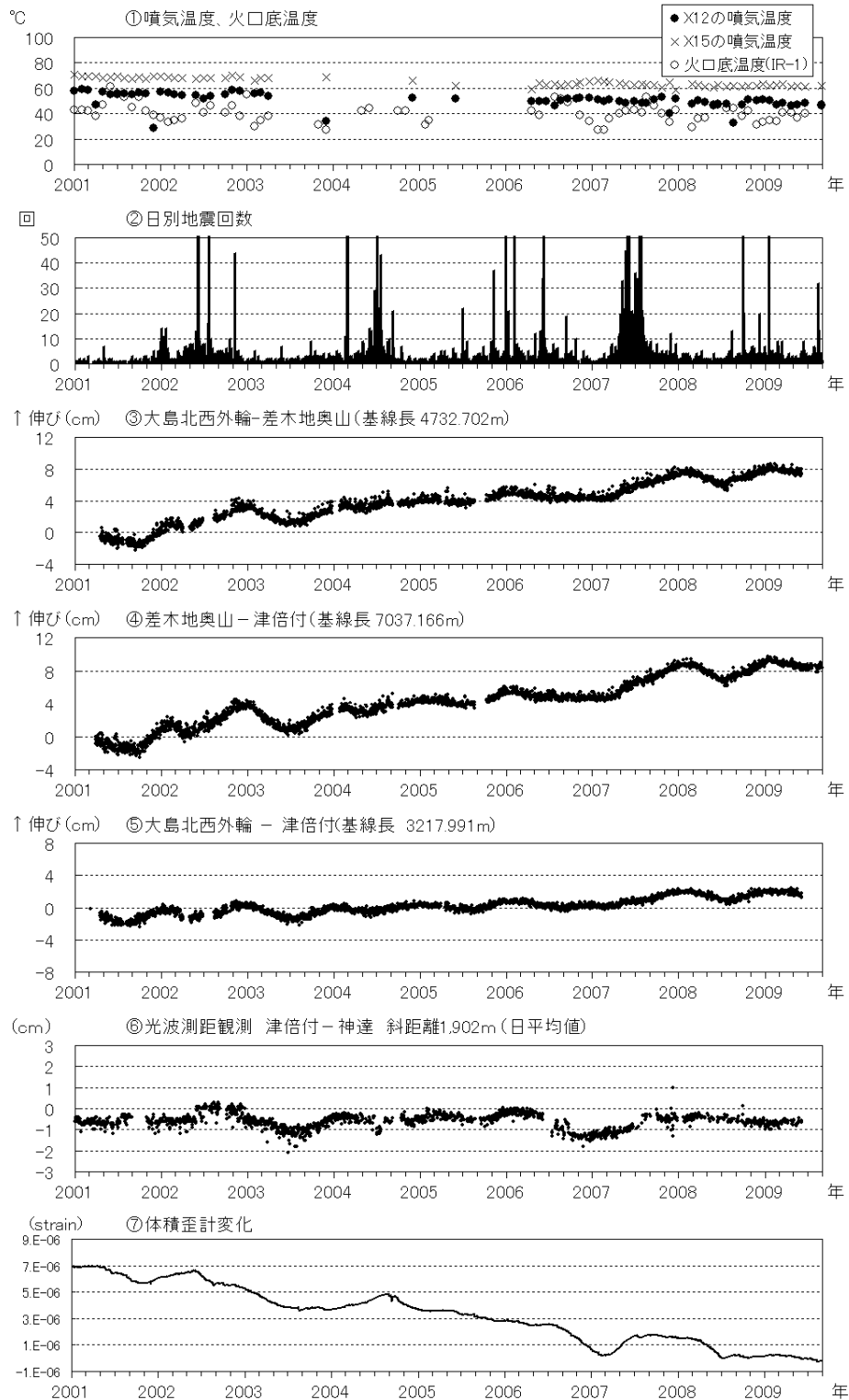
図5 伊豆大島 最近の火山活動経過図（2001年1月～2009年8月）
