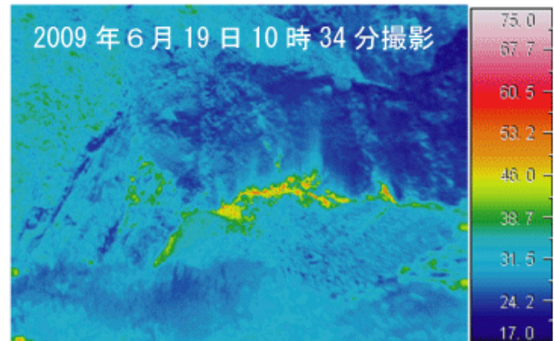
図1 伊豆大島 三原山山頂火口内及び山頂部の状況 右図の白円内は剣ガ峰付近のごく弱い噴気
