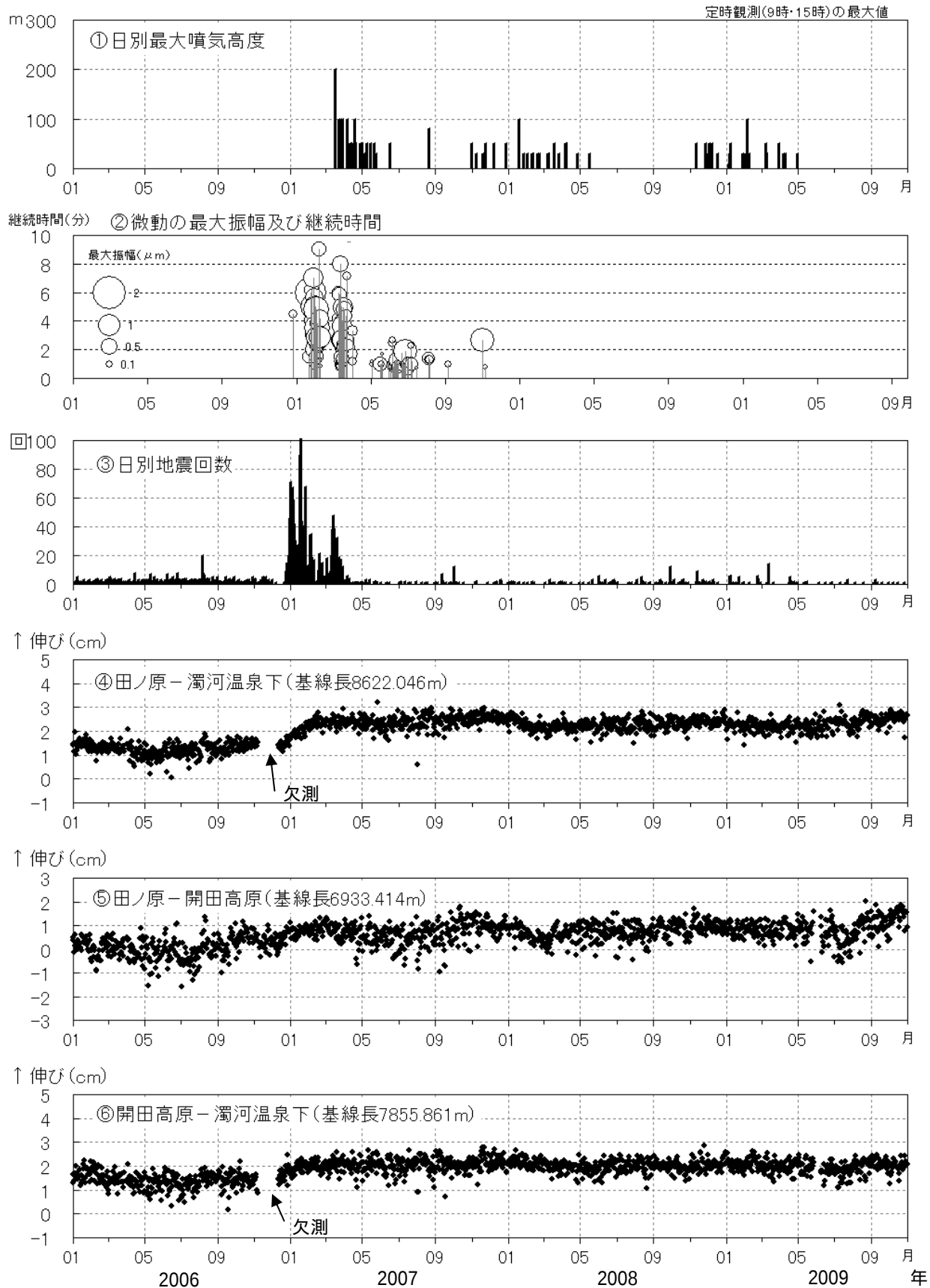
図2 御嶽山 最近の火山活動の推移（2006年1月1日～2009年10月31日）
