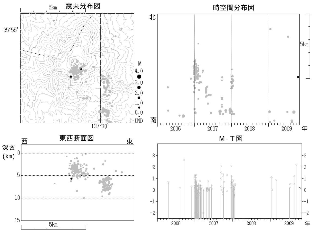
図 3 御嶽山 震源分布図（2006 年 1 月 1 日～2009 年 10 月 31 日）
