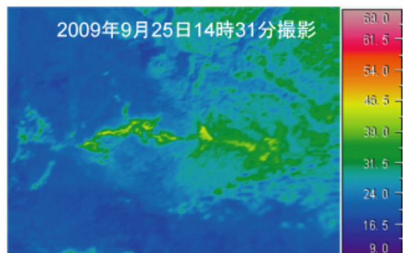
図 1 伊豆大島 三原山山頂火口内及び山頂部の状況 白円内は剣ガ峰付近のごく弱い噴気
