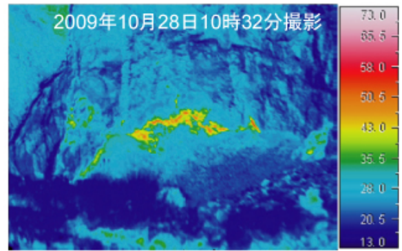
図 2 伊豆大島 中央火口内の状況（左）と地表面温度分布 1) （右）
