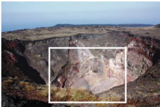
図 2 伊豆大島 中央火口内の状況（左）と地表面温度分布 1) （右）
