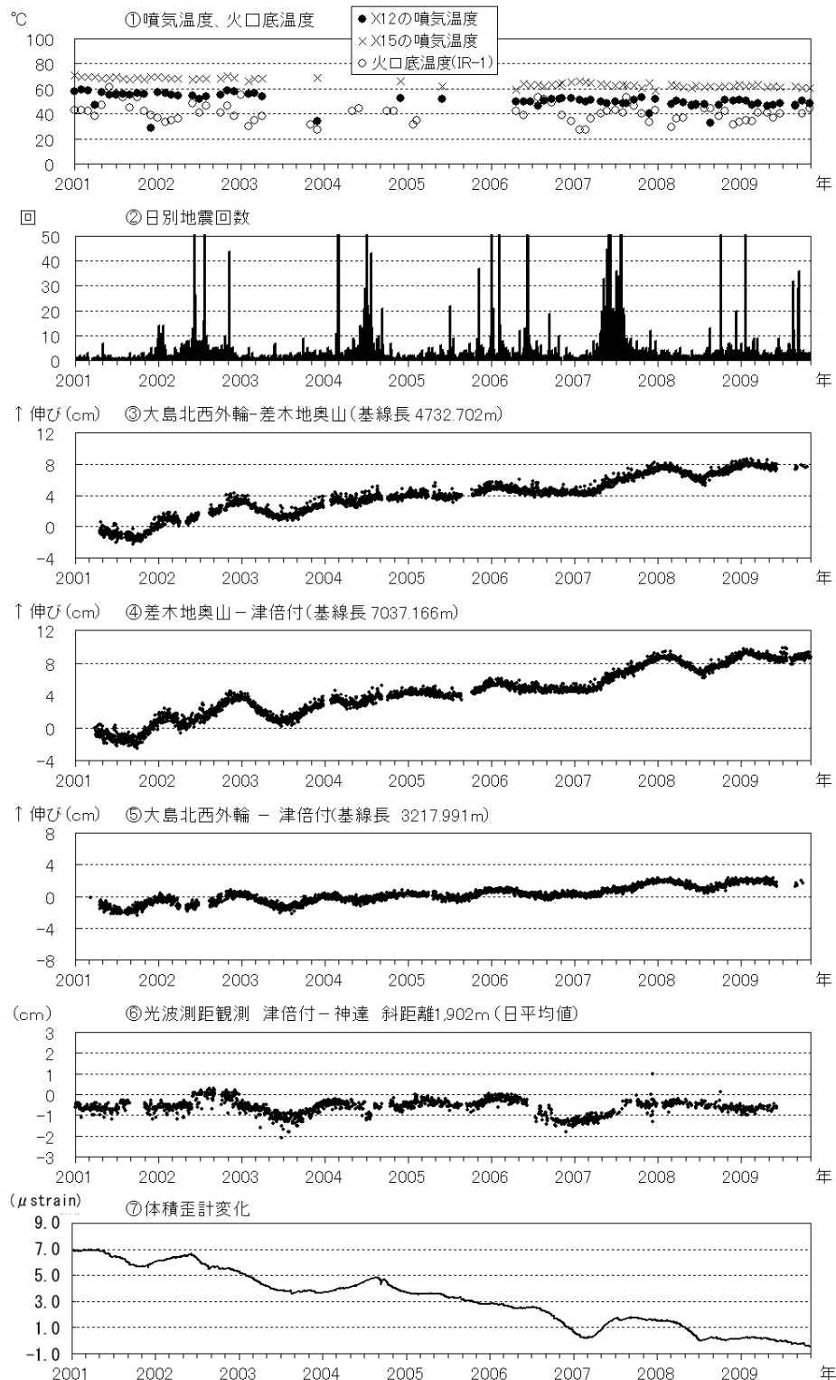
図5 伊豆大島 最近の火山活動経過図（2001年1月～2009年10月）
