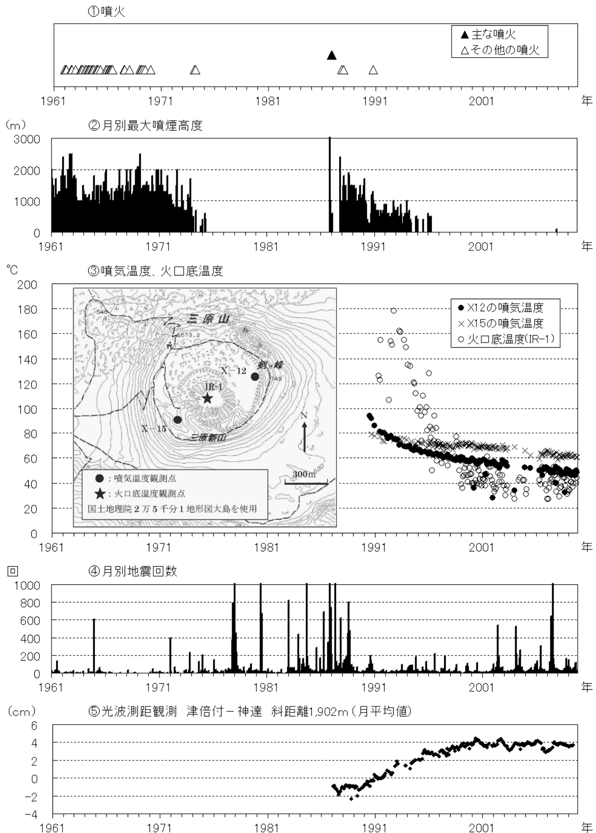
図4 伊豆大島 長期間の火山活動経過図（1961年1月～2009年10月）
