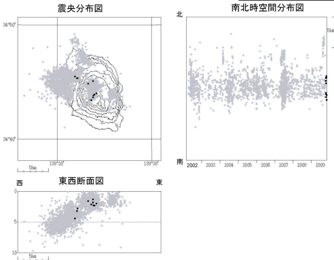
図 6 伊豆大島 震源分布図（2002 年 3 月 1 日 ~ 2009 年 10 月 31 日）
