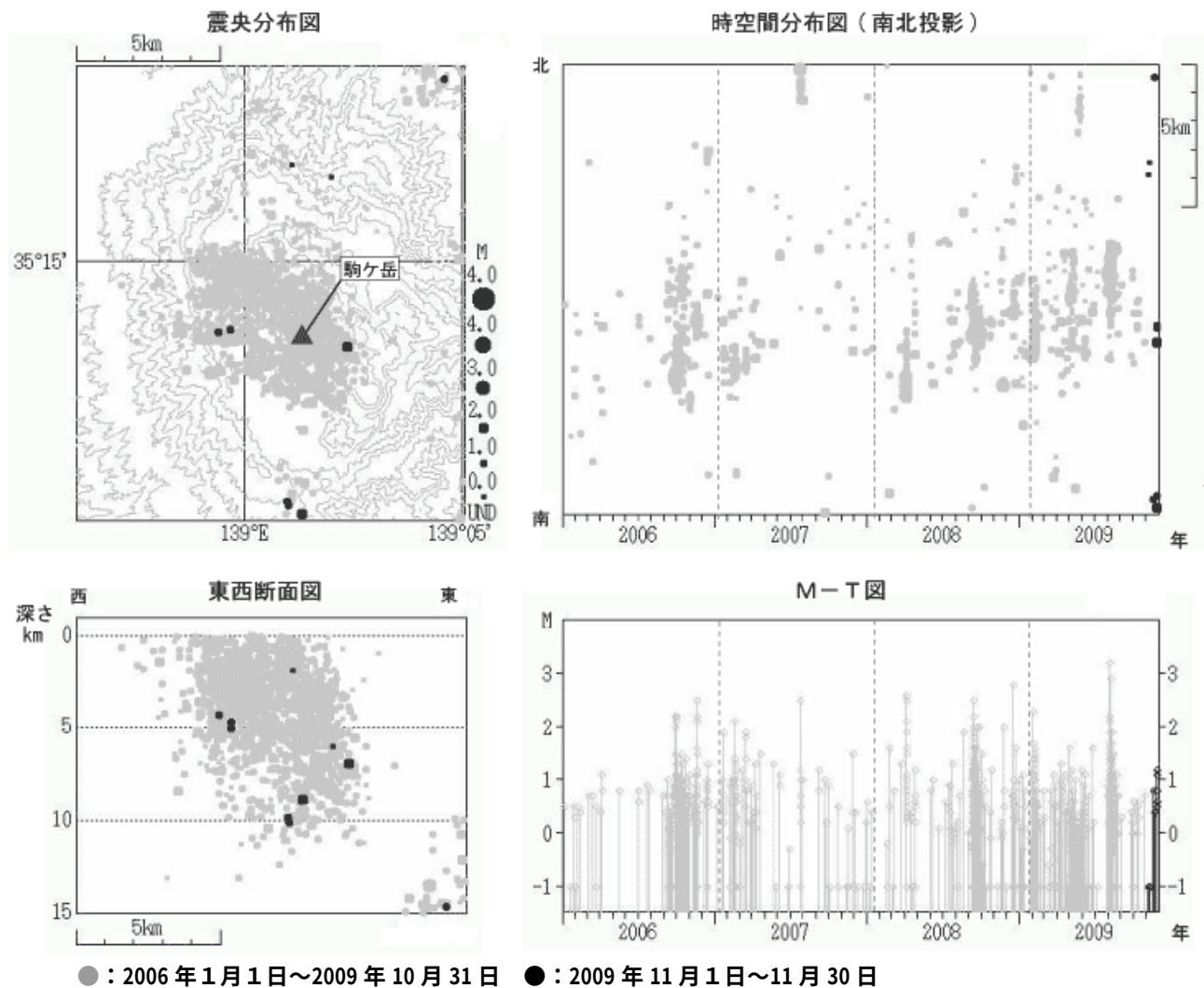
図 3 ※ 箱根山 震源分布図（2006 年 1 月 1 日～2009 年 11 月 30 日） M（マグニチュード）は地震の規模を表します。 図中の震源要素は一部暫定値が含まれており、後日変更することがあります。
