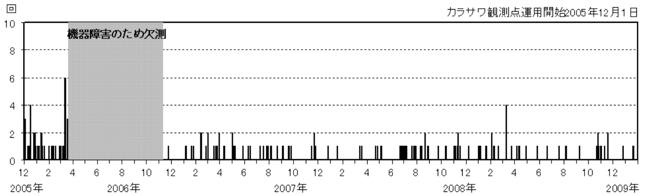
図2 新潟焼山 日別地震回数（2005年12月1日～2010年1月31日）
