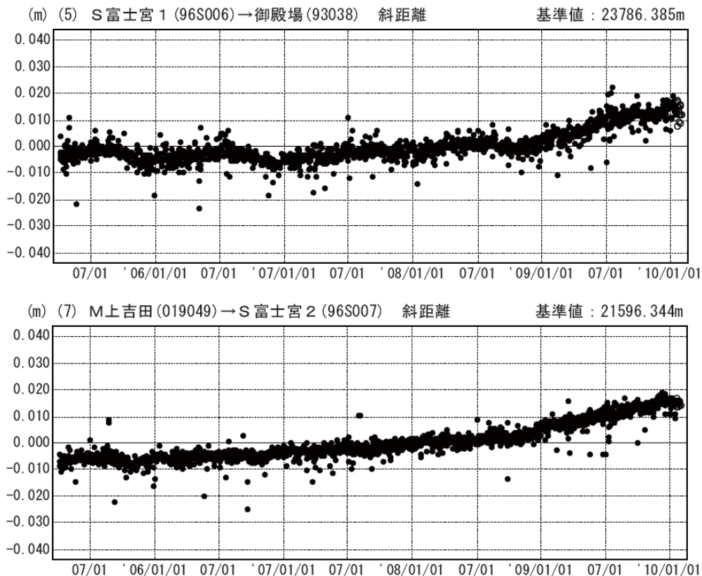
図 3 富士山 国土地理院による GPS 観測結果 1) (2005 年 4 月 1 日～2010 年 1 月 30 日)
