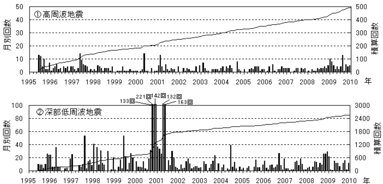
図 2 富士山 月別地震回数(1995 年 6 月～2010 年 1 月)
