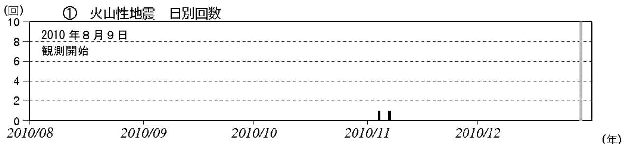
図 3 青ヶ島 火山性地震日別回数（2010 年 8 月 1 日～2010 年 12 月 31 日）
