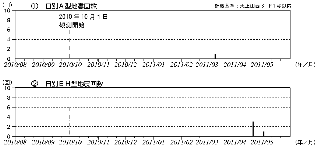
図 3 神津島 日別地震回数(2010 年 8 月～2011 年 5 月) 3 月～5 月分は一部未処理の期間があります。
