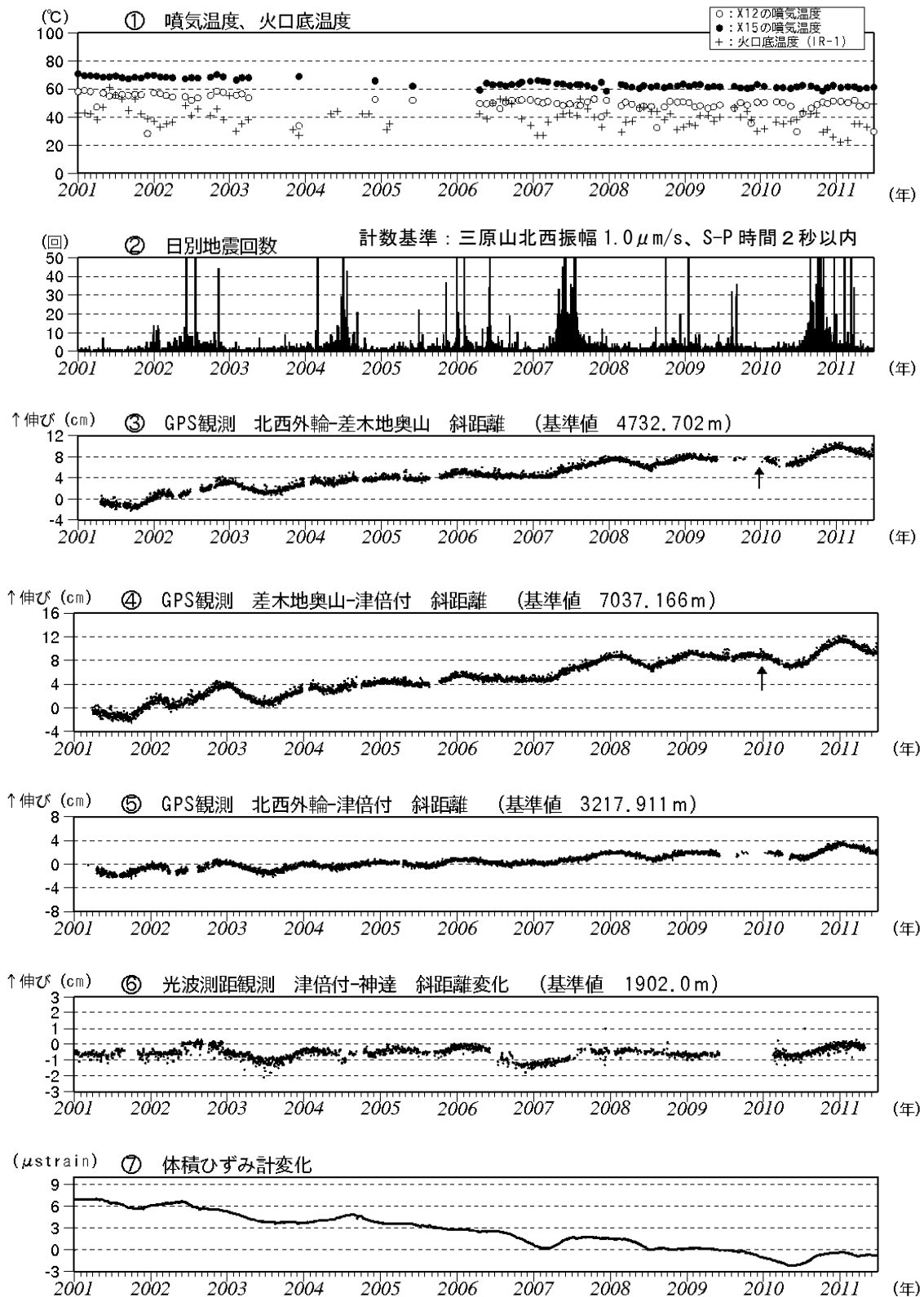
図2 伊豆大島 最近の火山活動経過図（2001年1月～2011年6月）
