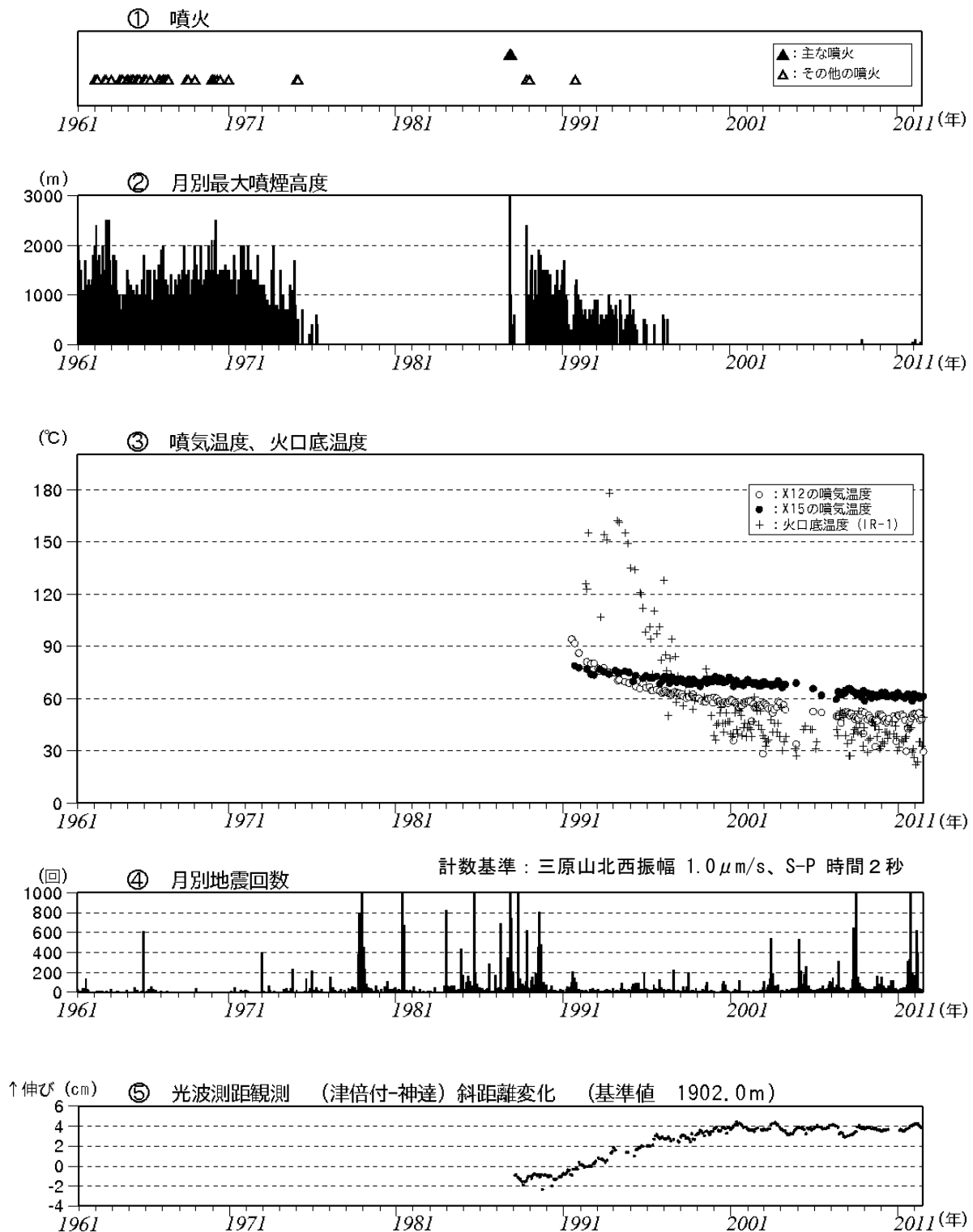
図 1 伊豆大島 長期間の火山活動経過図（1961 年 1 月～2011 年 6 月）
