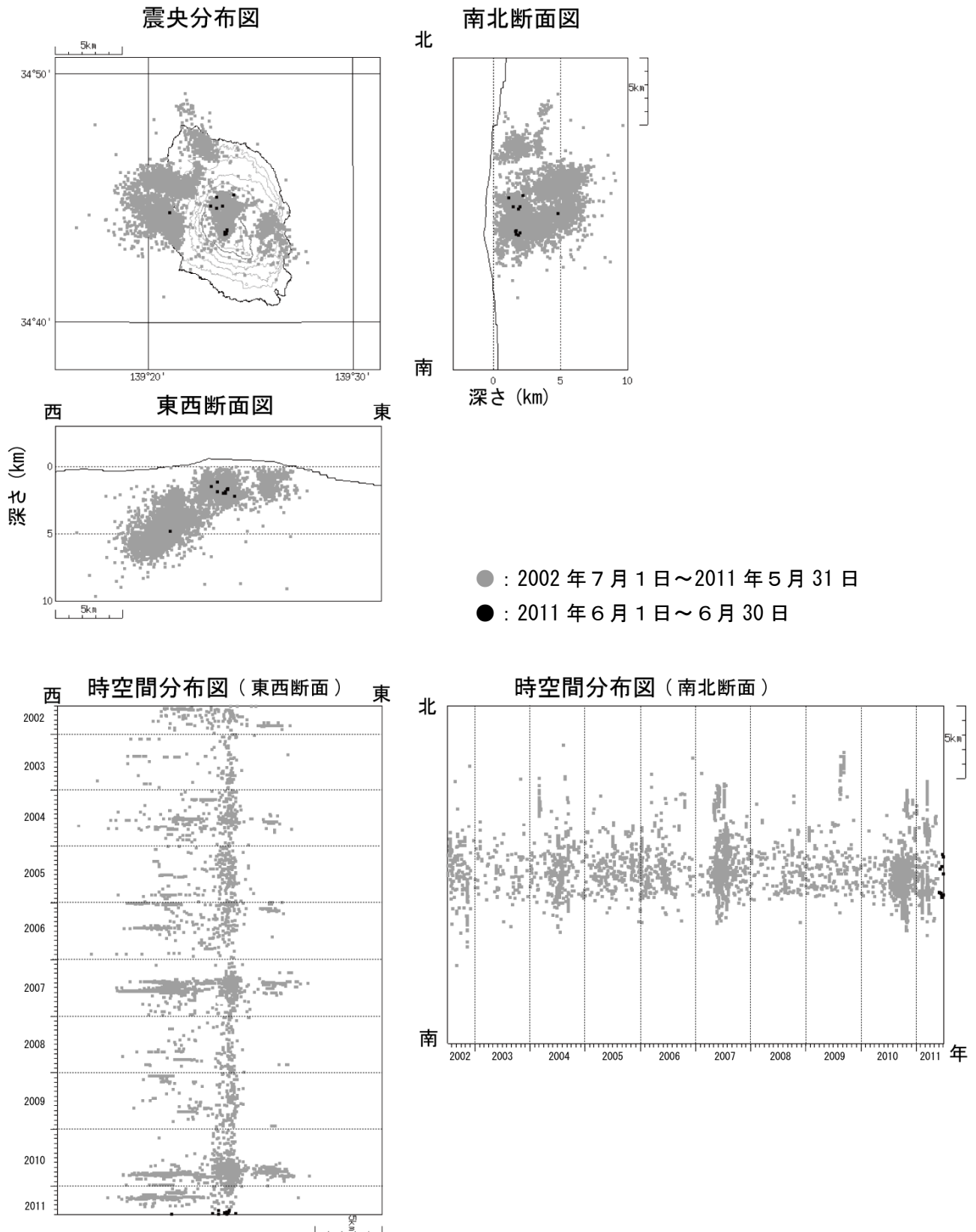
図 6※ 伊豆大島 震源分布図（2002 年 7 月 1 日～2011 年 6 月 30 日）
