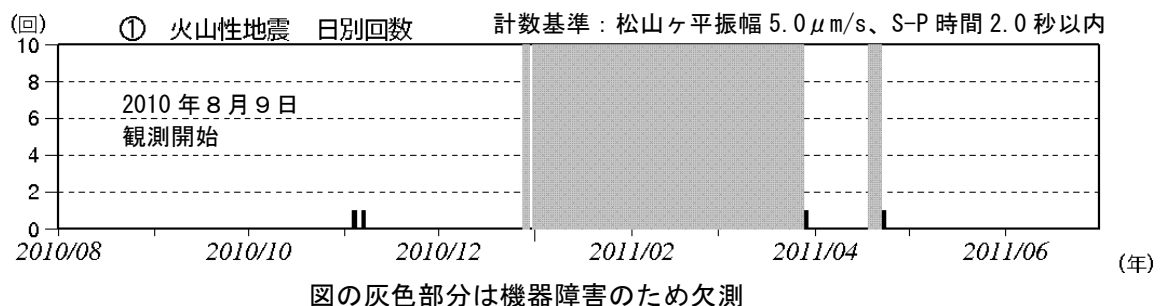
図 3 青ヶ島 火山性地震日別回数（2010 年 8 月 1 日～2011 年 6 月 30 日）
