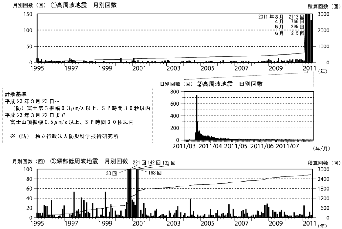
図 2 ※ 富士山 月別地震回数（1995 年 6 月～2011 年 7 月）
