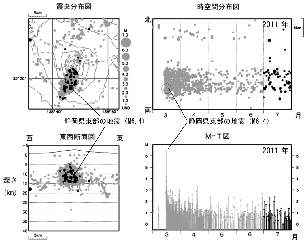
図 3 ※ 富士山 広域ネットによる山体・周辺の地震活動（1999 年 10 月 1 日～2011 年 7 月 31 日）
