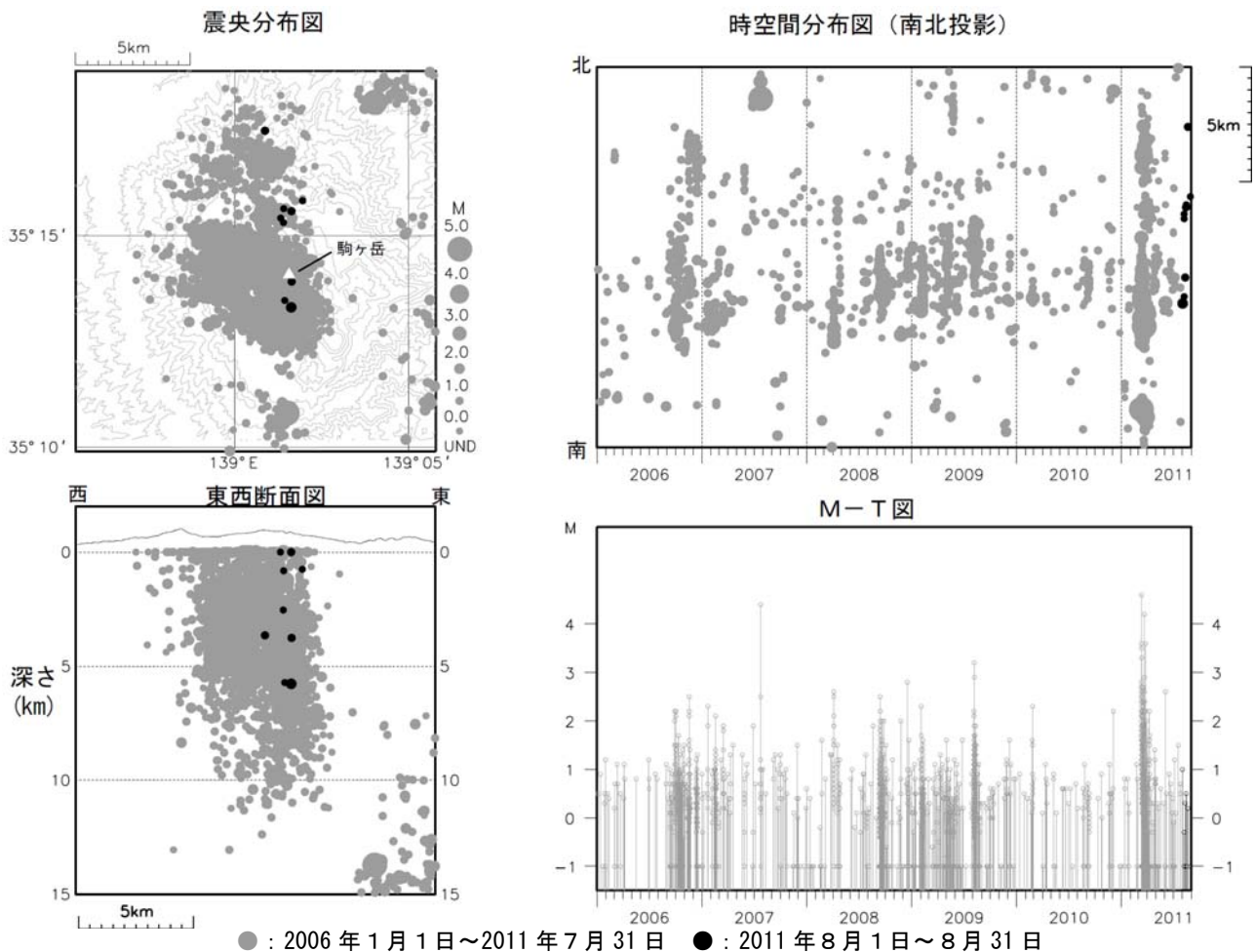
図 3※ 箱根山 広域ネットによる山体・周辺の震源分布図（2006 年 1 月 1 日～2011 年 8 月 31 日）
