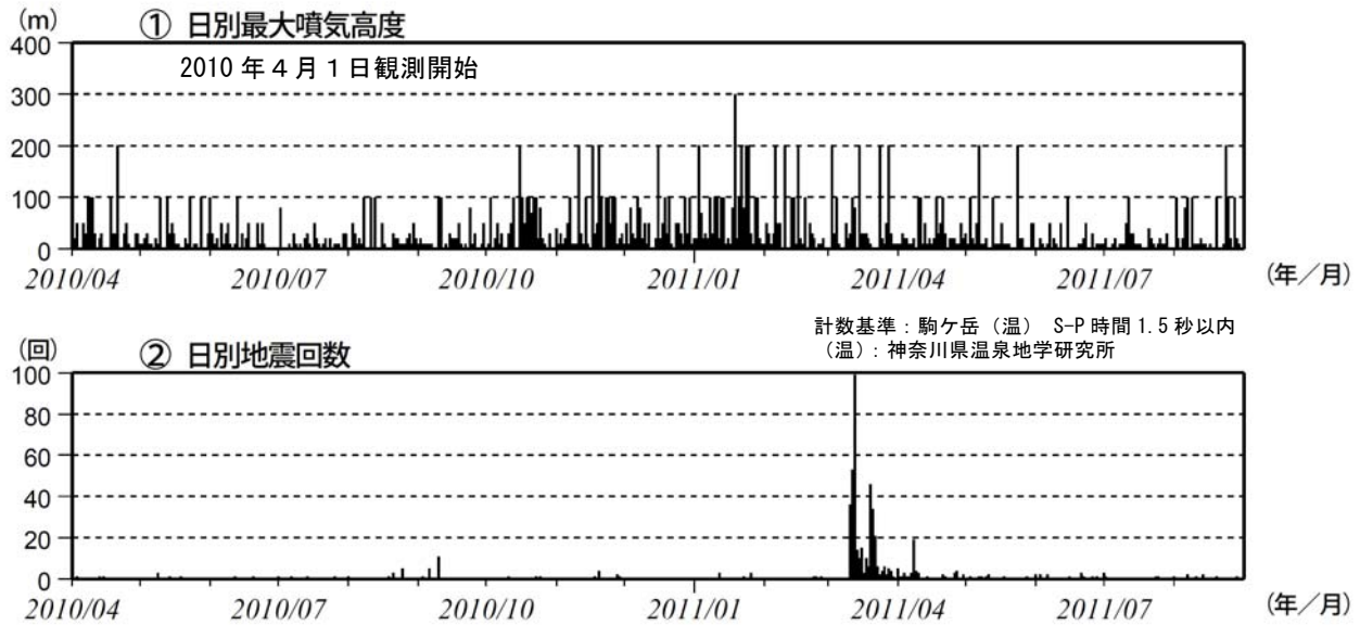
図 2※ 箱根山 火山活動の推移（2010 年 4 月 1 日～2011 年 8 月 31 日）
