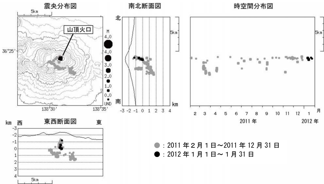
図 4 ※ 浅間山 震源分布図（2011 年 2 月 1 日～2012 年 1 月 31 日）
