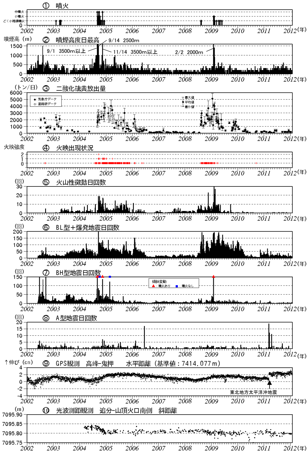
図 3 ※ 浅間山 最近の火山活動経過図（2002 年 1 月 1 日～2012 年 1 月 31 日）
