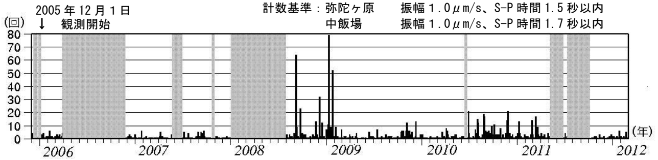
図 3 白山 日別地震回数（2005 年 12 月～2012 年 2 月）
