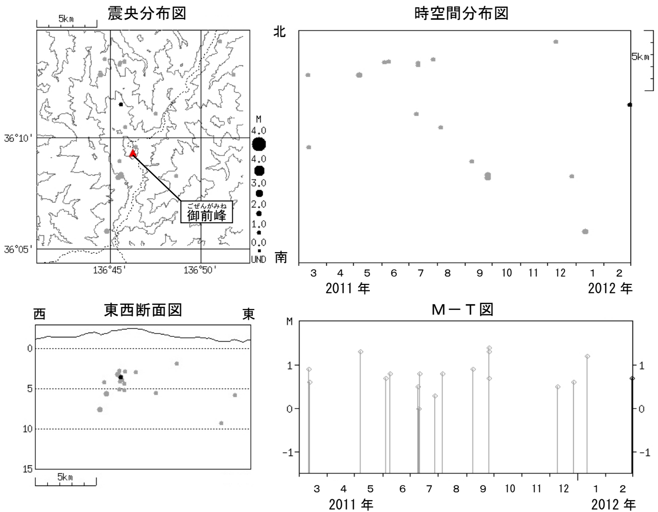
図 4 ※白山 広域地震観測網による山体・周辺の地震活動（2011 年 3 月～2012 年 2 月）
