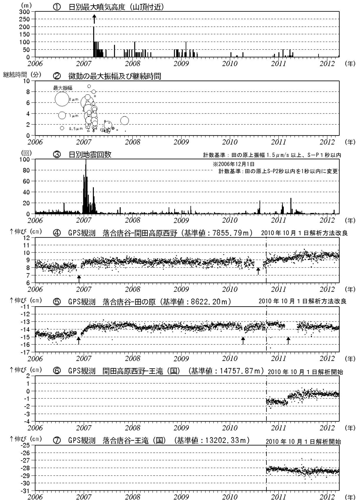
図3 御嶽山 最近の火山活動経過図（2006年1月1日～2012年3月31日）
