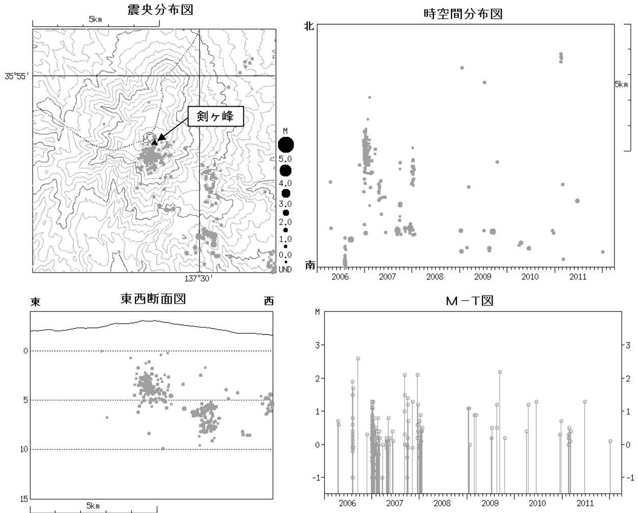
図 4 ※ 御嶽山 広域地震観測網による山体・周辺の震源分布図（2006 年 1 月 1 日～2012 年 3 月 31 日）
