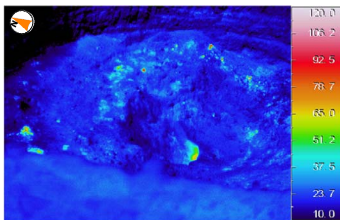
図 3 浅間山 山頂火口の状況及び赤外熱映像装置 1) による地表面温度分布
