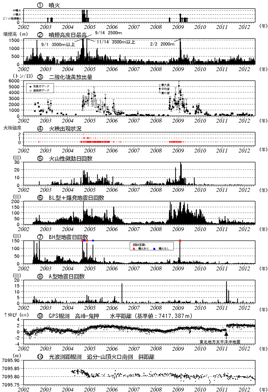
図5※ 浅間山 最近の火山活動経過図（2002年1月1日～2012年6月30日）
