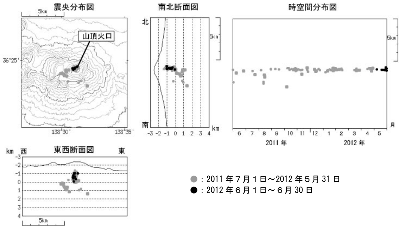
図 6※ 浅間山 震源分布図（2011 年 7 月 1 日～2012 年 6 月 30 日）
