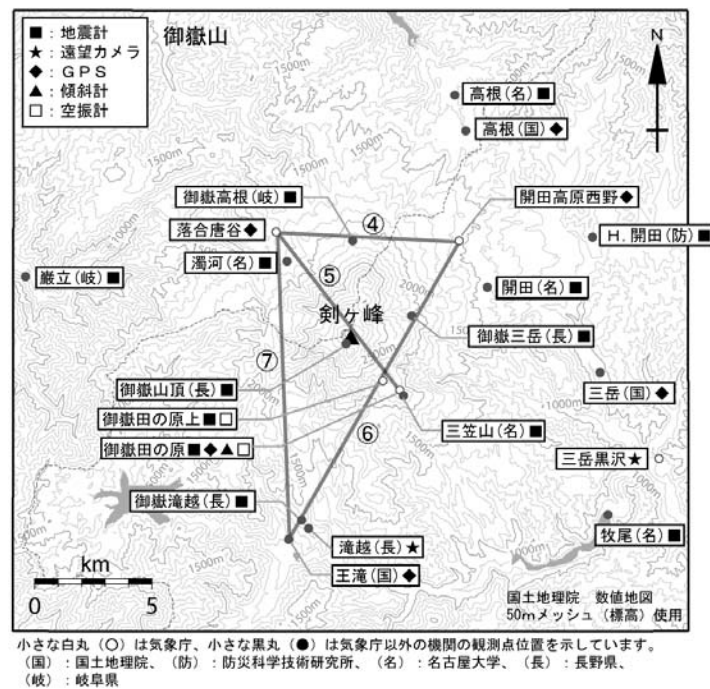
図 5 御嶽山 観測点配置図
