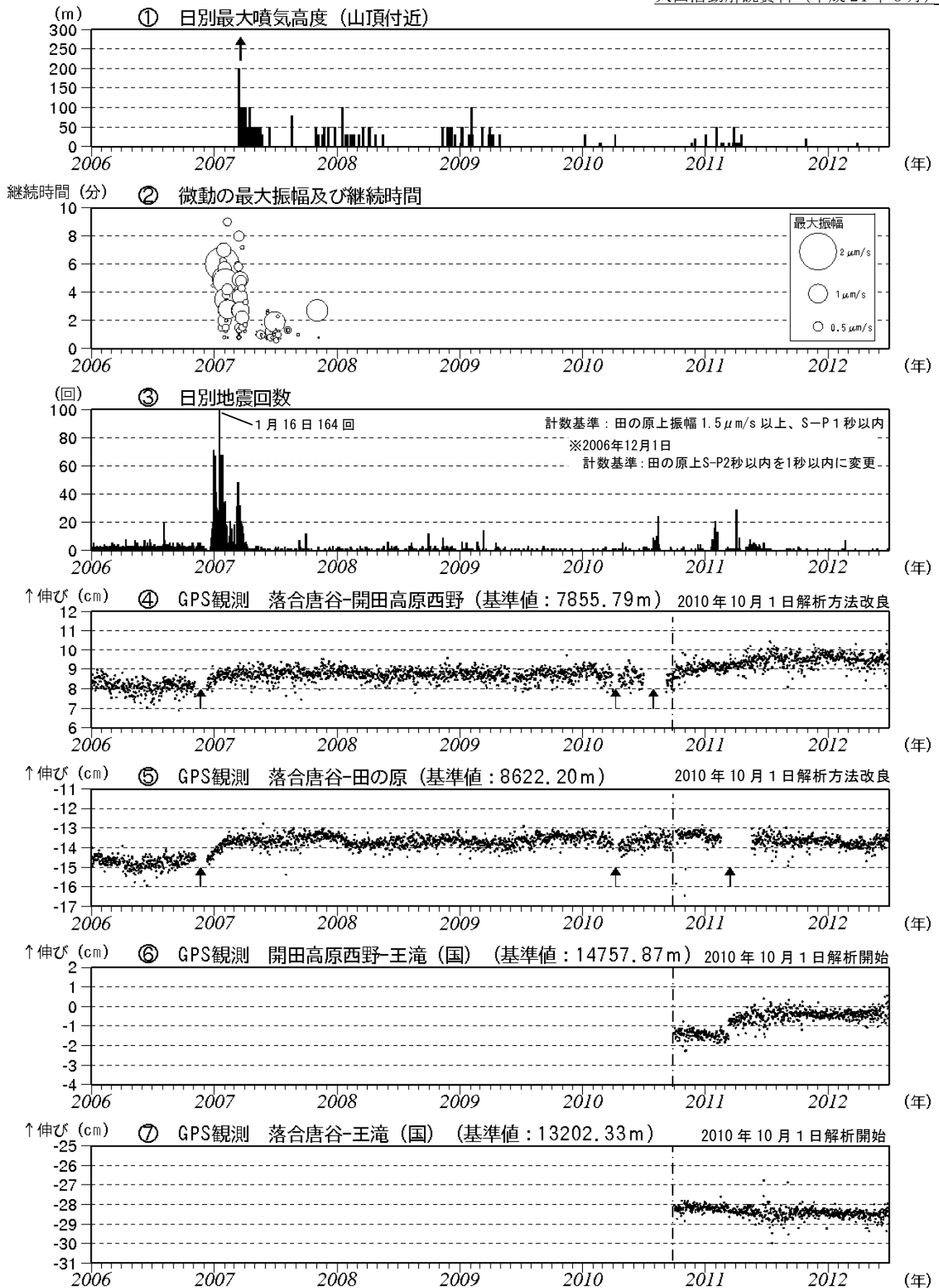
図3 御嶽山 最近の火山活動経過図（2006年1月1日～2012年6月30日）
