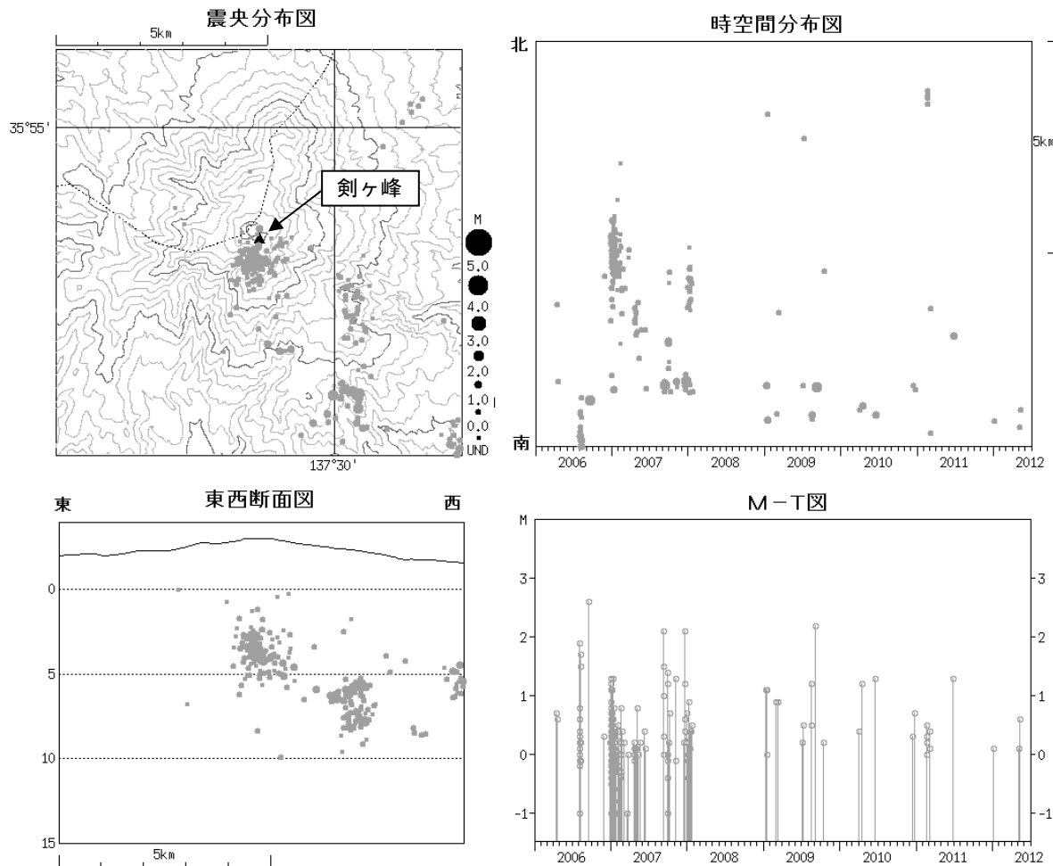
図 4 ※ 御嶽山 広域地震観測網による山体・周辺の震源分布図（2006 年 1 月 1 日～2012 年 6 月 30 日）
