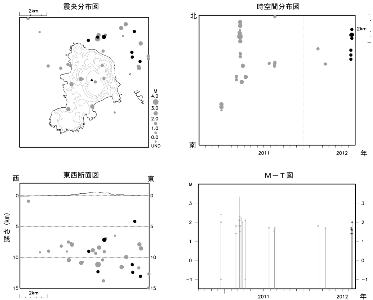
図 4 ※ 神津島 広域地震観測網による山体・周辺の地震活動（2010 年 9 月 1 日～2012 年 8 月 31 日）
