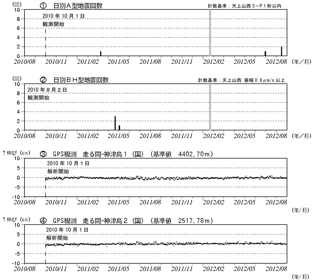
図 3 神津島 火山活動経過図(2010 年 8 月 2 日~2012 年 8 月 31 日) ①②神津島周辺の日別地震回数 図の灰色部分は機器障害のため欠測。 ③※④※ GPS 連続観測による基線長変化 (国)：国土地理院 ③※④※は図 1 の GPS 基線③④に対応しています。
