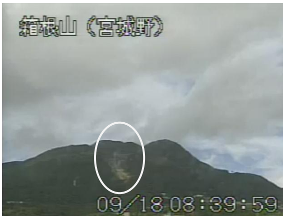
図 1 箱根山 早雲地獄の状況
