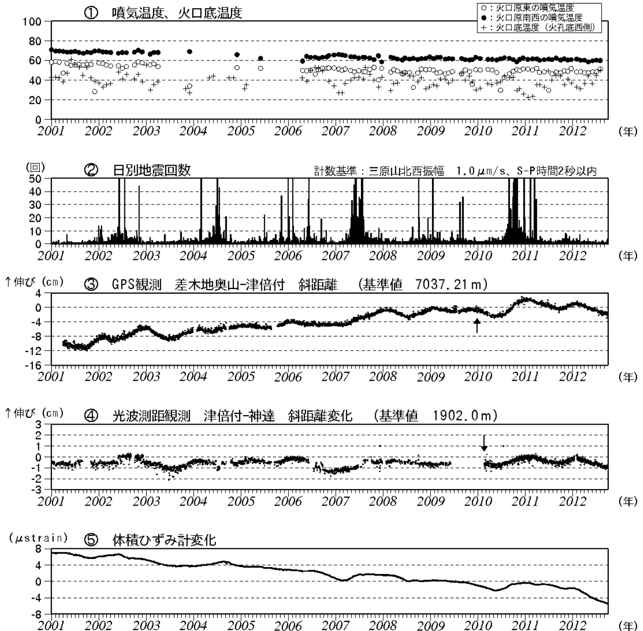
図2 伊豆大島 最近の火山活動経過図（2001年1月～2012年9月）
