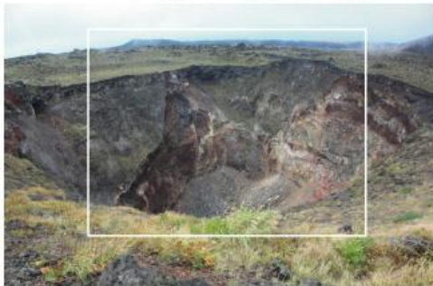
2012年10月4日の火口内の画像
