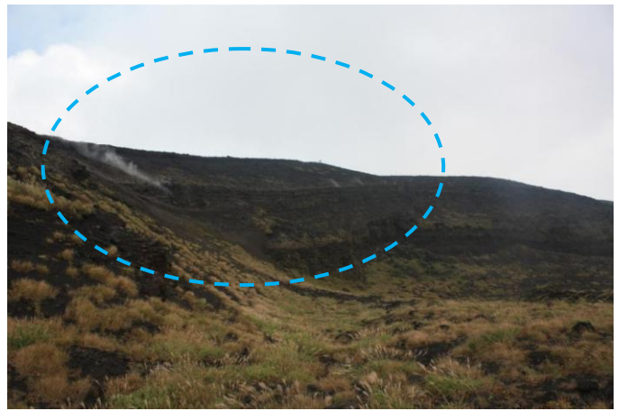
山頂部（9月24日、北西外輪遠望カメラによる） 剣ガ峰付近（10月4日、撮影方向は図6参照） 図4 伊豆大島 三原山山頂部及び山頂火口の状況 点円内：ごく弱い噴気
