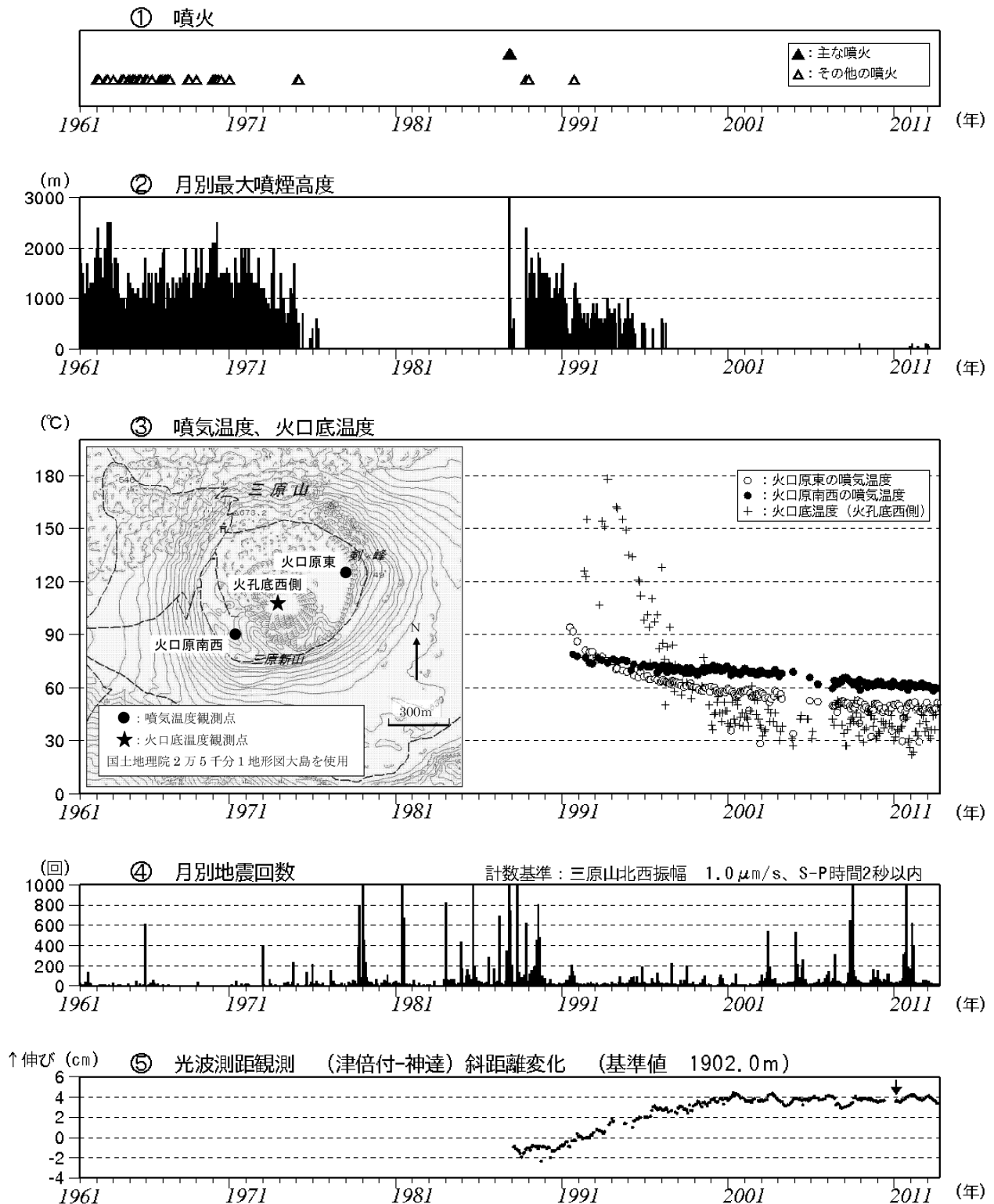
図 1 伊豆大島 長期間の火山活動経過図（1961 年 1 月～2012 年 9 月）
