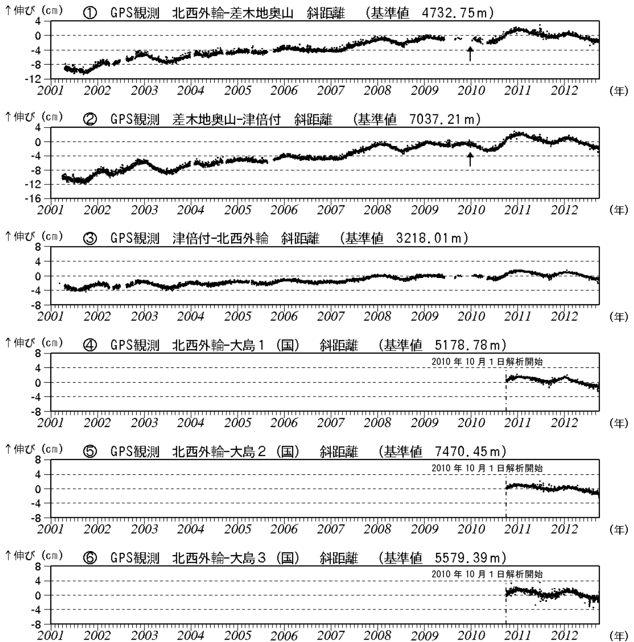
図3※ 伊豆大島 GPS 連続観測による基線長変化 (2001 年 1 月～2012 年 9 月) (国) : 国土地理院 2010 年 10 月以降のデータについては、電離層の影響を補正する等、解析方法を改良しています。 ①～③、及び④※～⑥※は図8のGPS基線①～⑥に対応しています。 グラフの空白部分は欠測。①②の矢印は差木地奥山支柱工事による変動。
