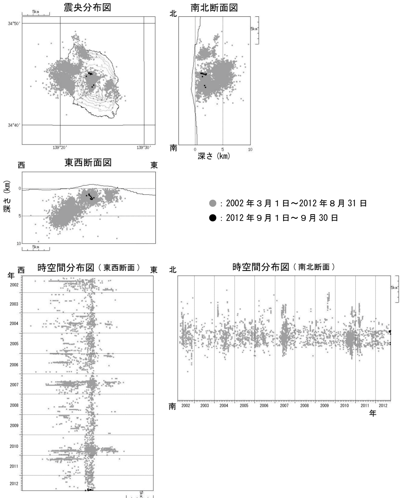
図 7 ※ 伊豆大島 震源分布図（2002 年 3 月 1 日～2012 年 9 月 30 日）
