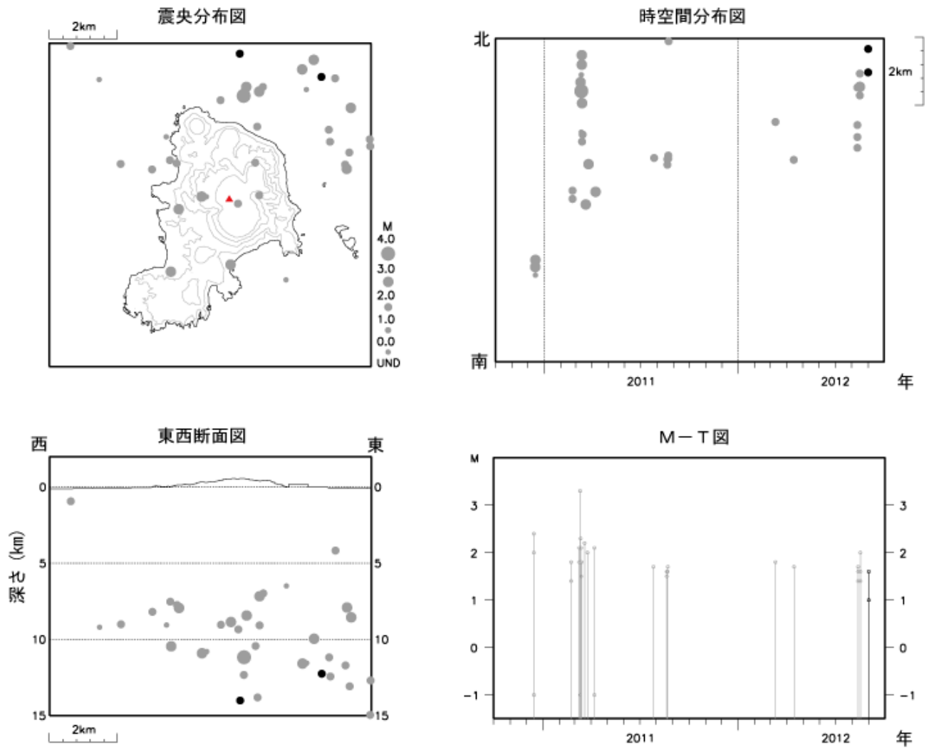
図 4※ 神津島 広域地震観測網による山体・周辺の地震活動（2010 年 10 月 1 日～2012 年 9 月 30 日）
