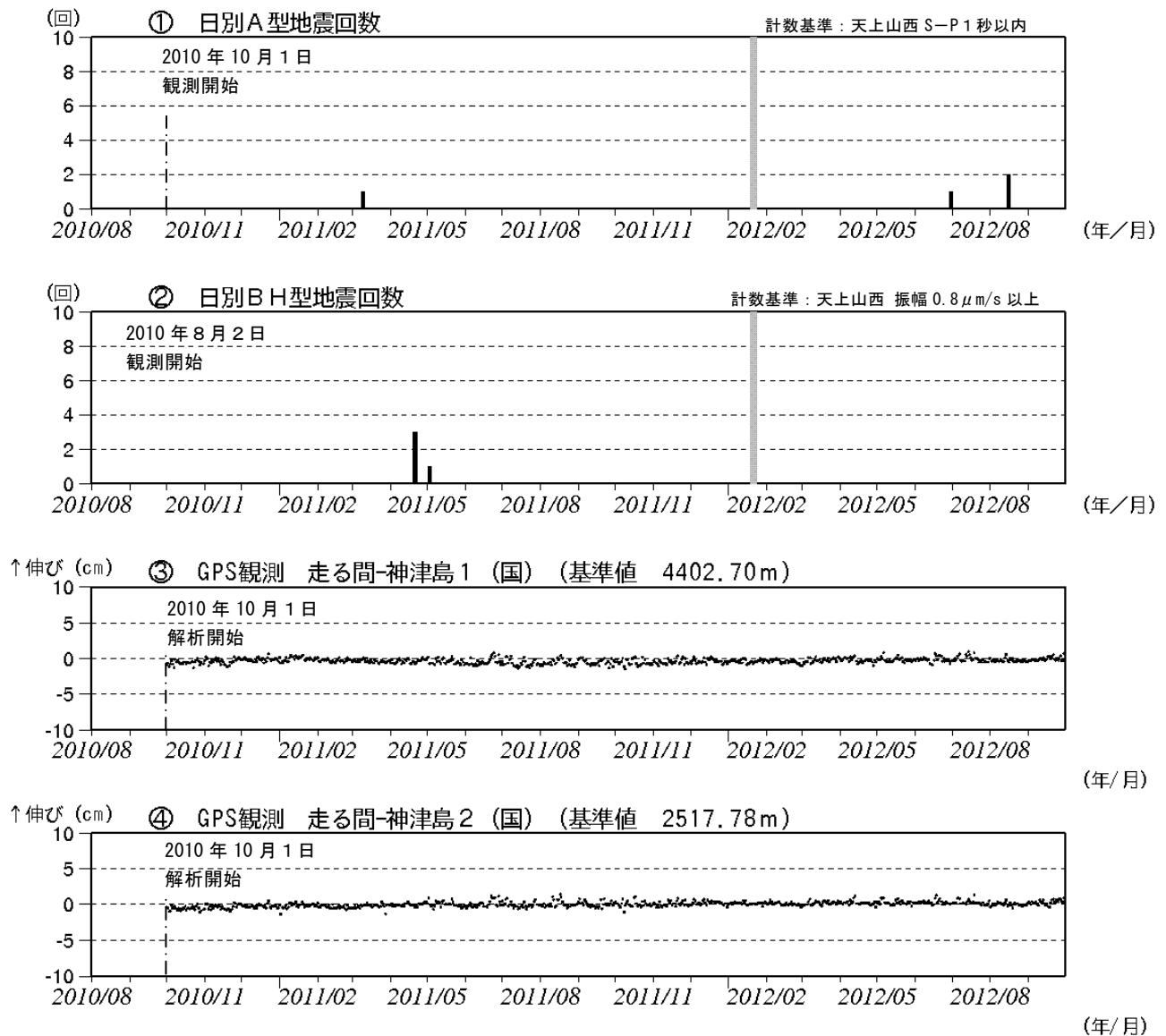
図3 神津島 火山活動経過図(2010 年 8 月 2 日~2012 年 9 月 30 日) ①②神津島周辺の日別地震回数 図の灰色部分は機器障害のため欠測。 ③※④※ GPS 連続観測による基線長変化 (国)：国土地理院 ③※④※は図1のGPS基線③④に対応しています。
