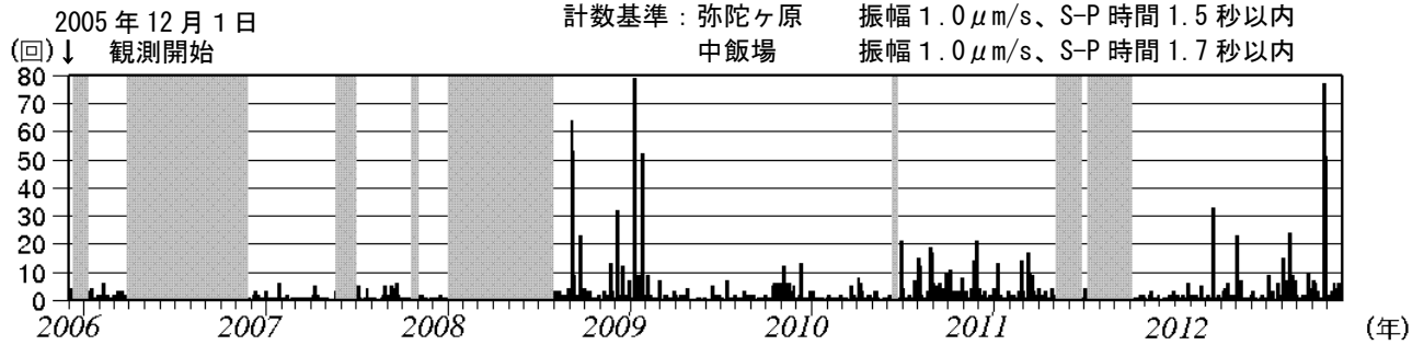
図 3 白山 日別地震回数（2005 年 12 月～2012 年 11 月）
