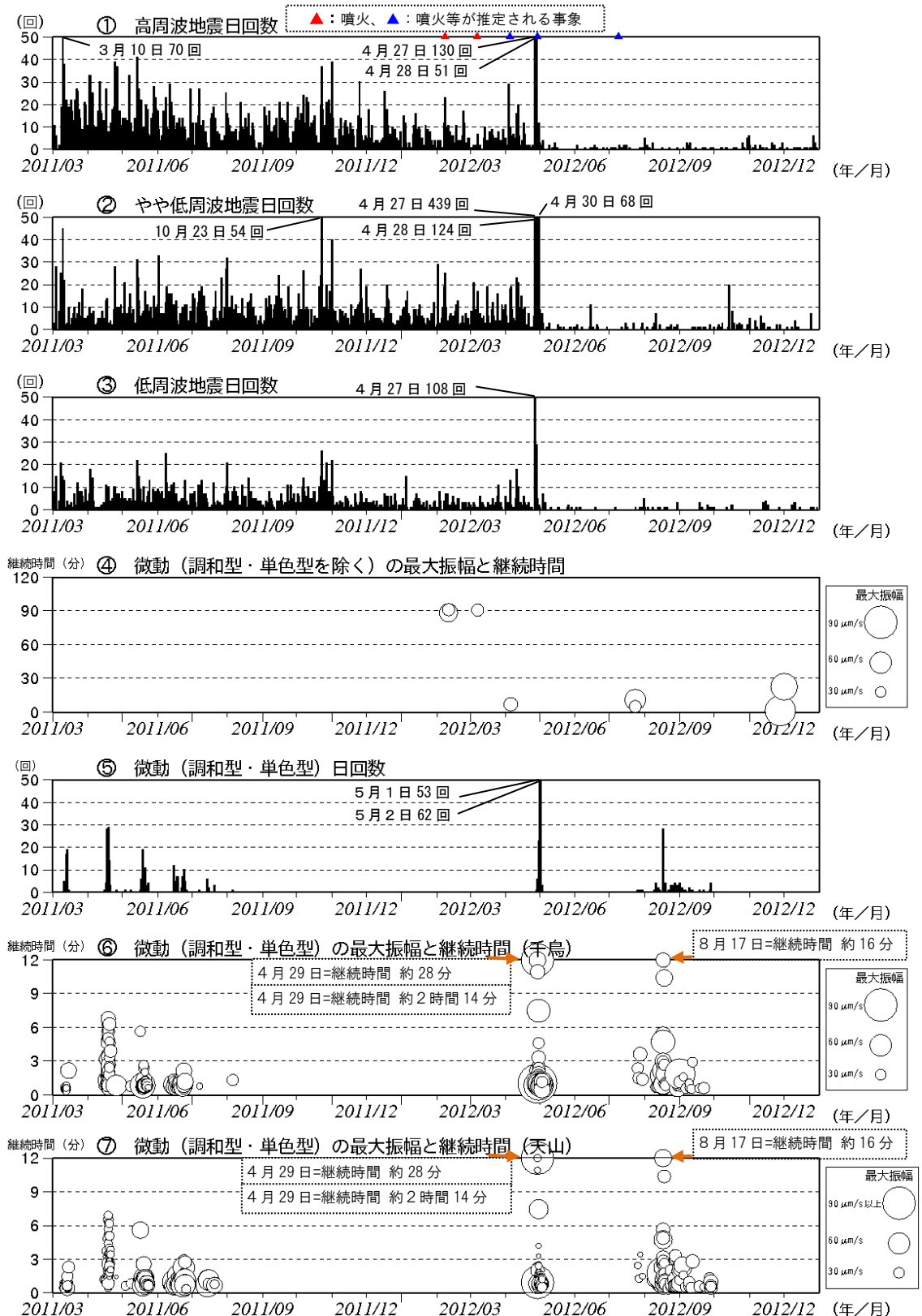
図 5 ※ 硫黄島 火山活動経過図（2011 年 3 月 8 日～2012 年 12 月 31 日）
