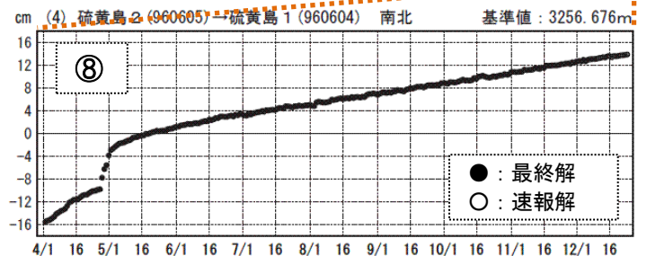
図 6※ 硫黄島 国土地理院による地殻変動観測結果 1) (2008 年 1 月 1 日～2012 年 12 月 23 日)
