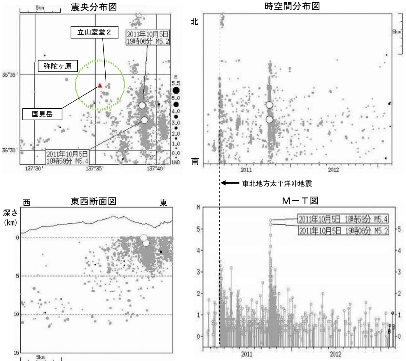
図 2※ 弥陀ヶ原 広域地震観測網による山体・周辺の地震活動（2011 年 1 月 1 日～2013 年 2 月 28 日）
