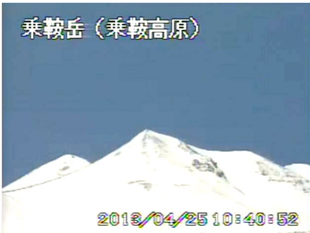
図 1 乗鞍岳 山頂部の状況 （4 月 25 日 乗鞍高原遠望カメラによる）
