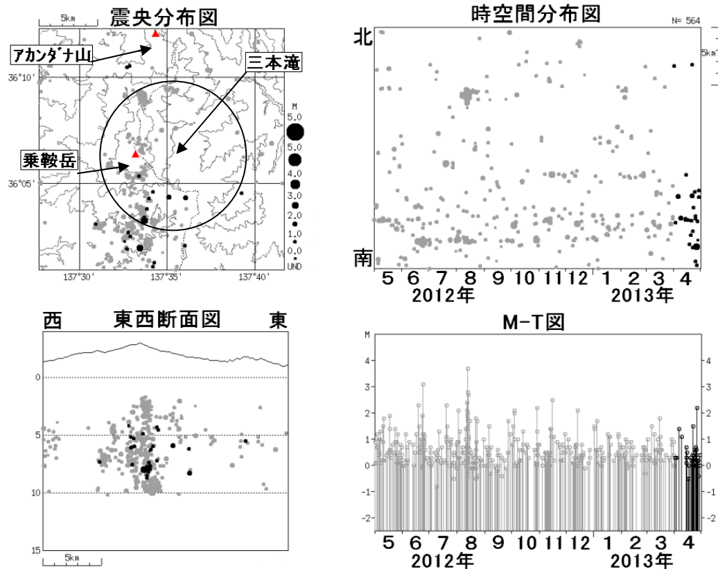
図 3 ※ 乗鞍岳 広域地震観測網による山体・周辺の地震活動(2012 年 5 月～2013 年 4 月) ● : 2012 年 4 月 1 日～2013 年 3 月 31 日 ● : 2013 年 4 月 1 日～4 月 30 日 震央分布図中の円は図 2 の計数対象地震（三本滝で S-P 時間 1 秒以内）のおよその範囲。 M（マグニチュード）は地震の規模を表します。 図中の震源要素は一部暫定値が含まれており、後日変更することがあります。
